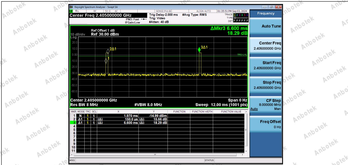
NTNV-2.4G-Ant1-2405
