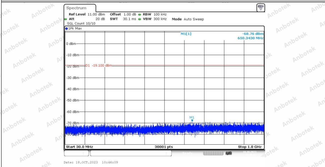
2.4G_Ant1_2441_30~1000
