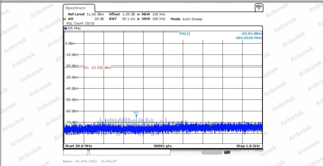
2.4G_Ant1_2442_30~1000
