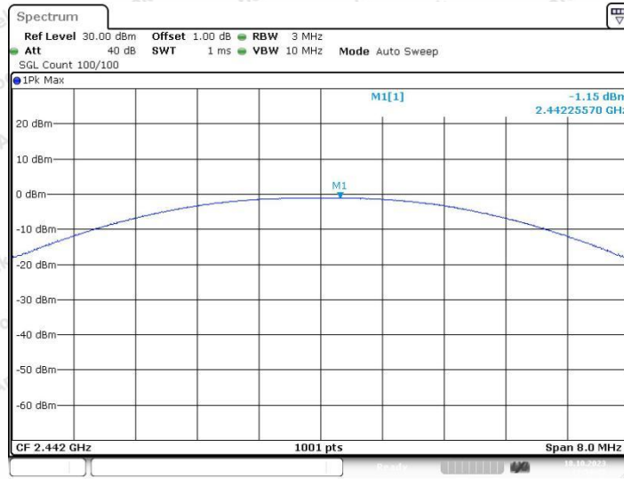
2.4G_Ant1_2442
