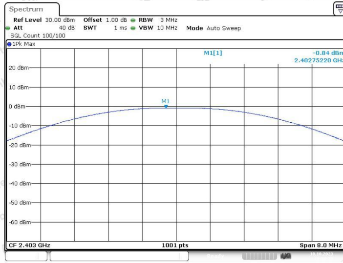
2.4G_Ant1_2403
