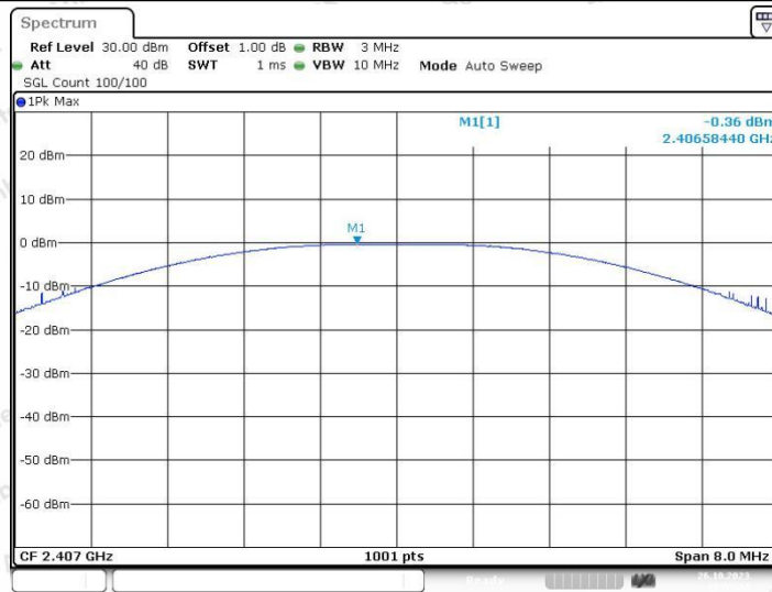
2.4G_Ant1_2407
