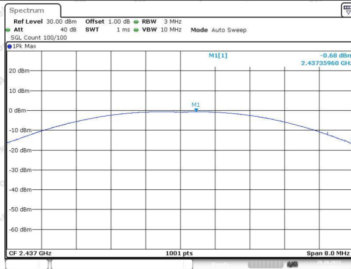
2.4G_Ant1_2437
