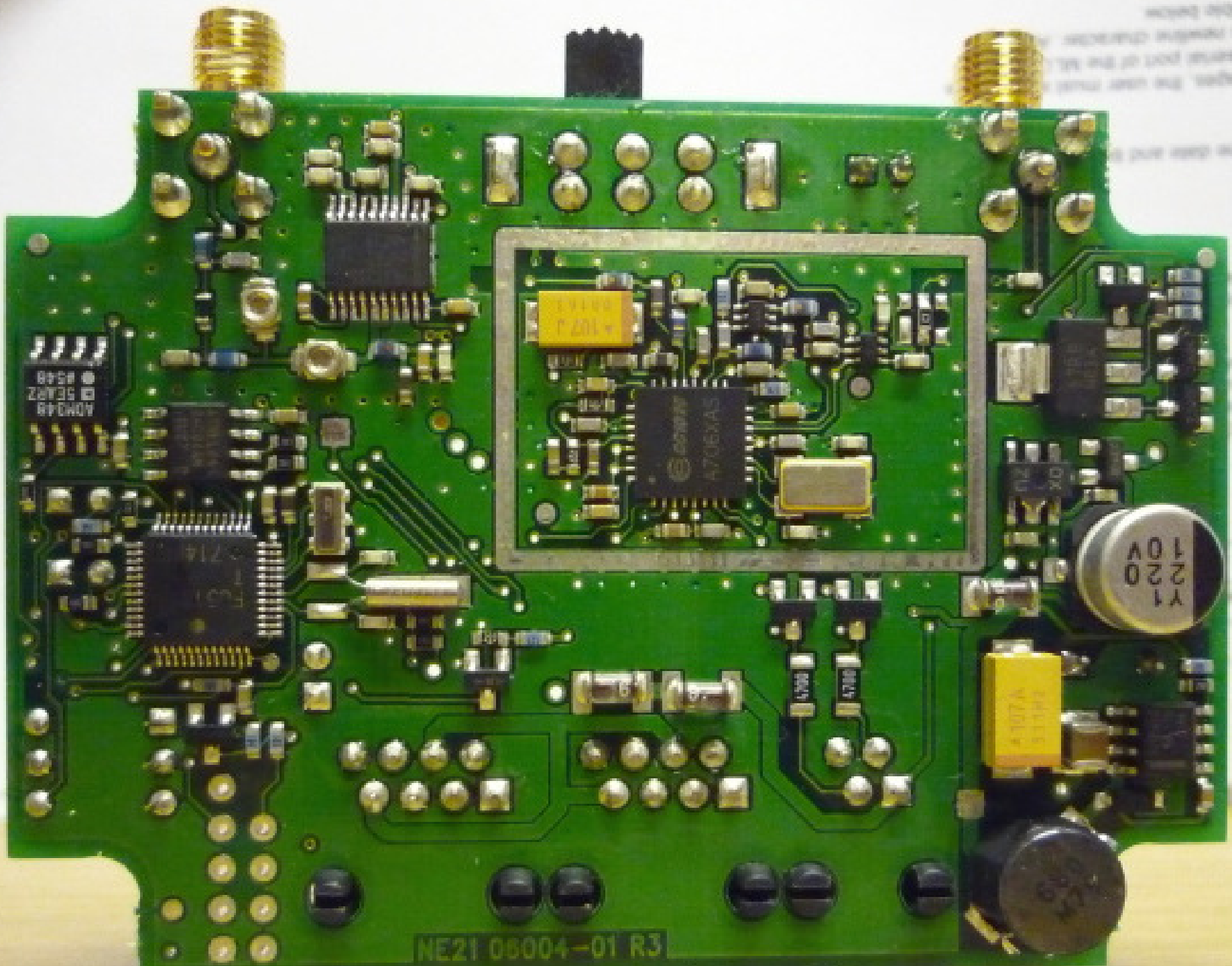
D-TECT-PCB-back
