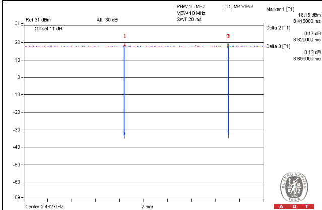
802.11n (HT20)
