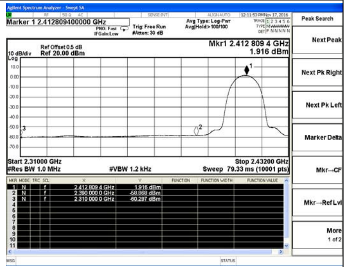
802.11b-Low channel(Average)
