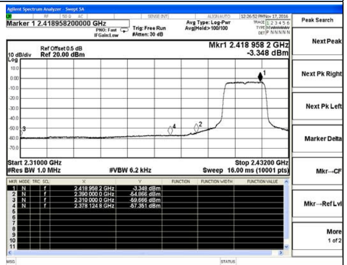
802.11n(HT20)-Low channel(Average)
