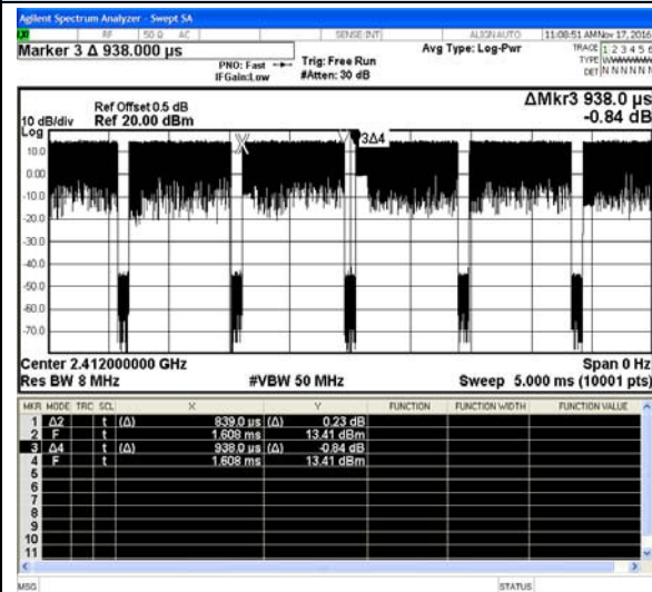
IEEE 802.11b
