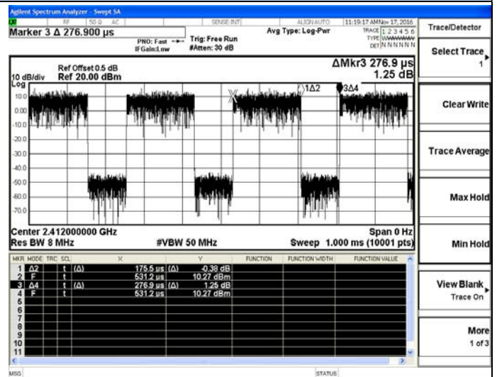
IEEE 802.11g
