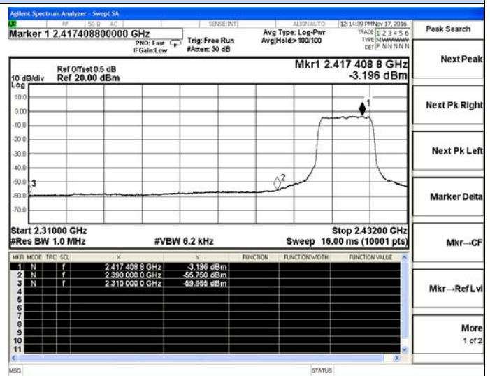
802.11g-Low channel(Average)
