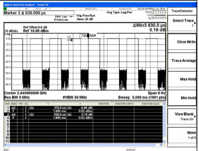
BT LE
