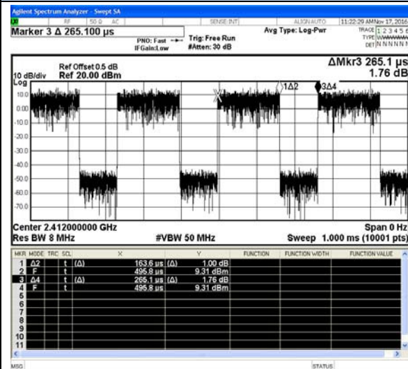
IEEE 802.11n-HT20
