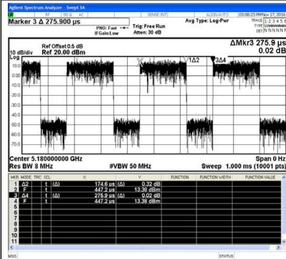
IEEE 802.11a
