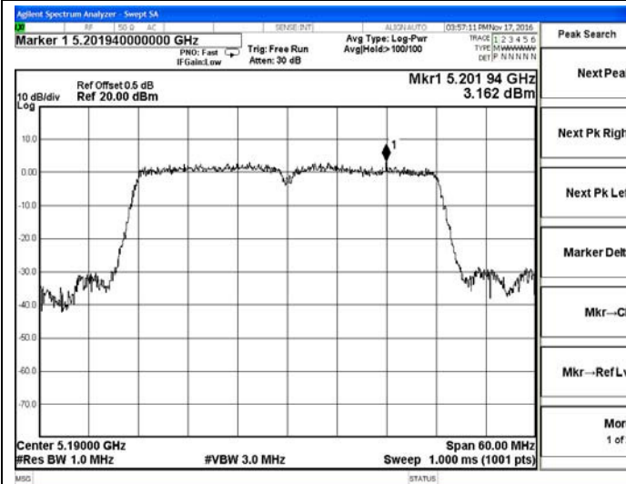
IEEE 802.11n-HT40-5190MHz
