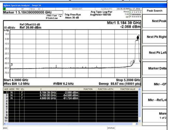
802.11n-HT20-Low channel(Average)
