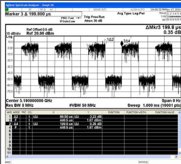
IEEE 802.11n-HT40
