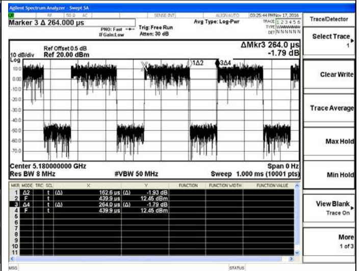
IEEE 802.11n-HT20
