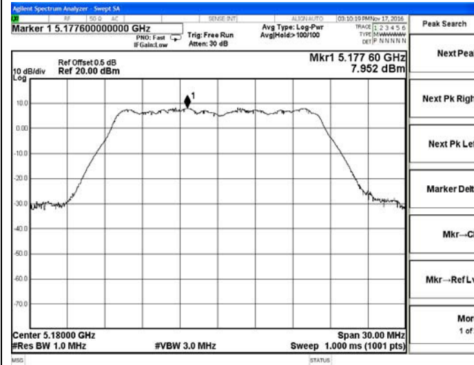
IEEE 802.11a-5180MHz
