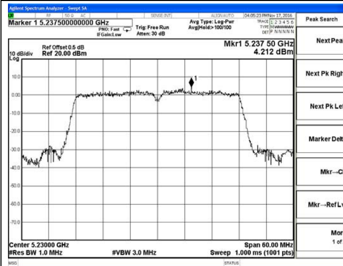
IEEE 802.11n-HT40-5230MHz
