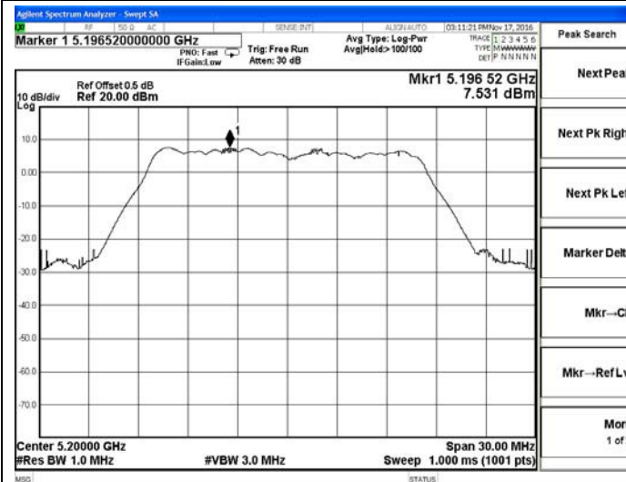
IEEE 802.11a-5200MHz
