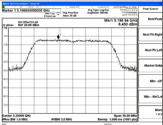
IEEE 802.11n-HT20-5200MHz
