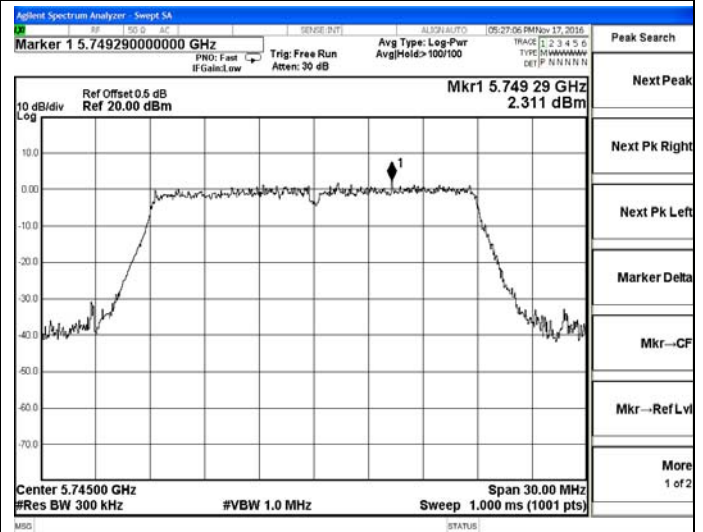
IEEE 802.11ac VHT20-5745MHz
