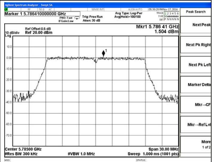
IEEE 802.11ac VHT20-5785MHz
