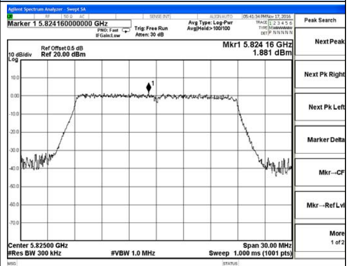
IEEE 802.11ac VHT20-5825MHz
