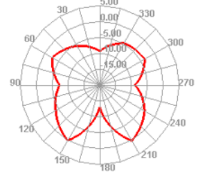
2450.000MHz E2
