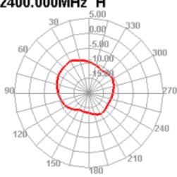
2400.000MHz H
