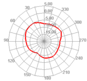
2450.000MHz H
