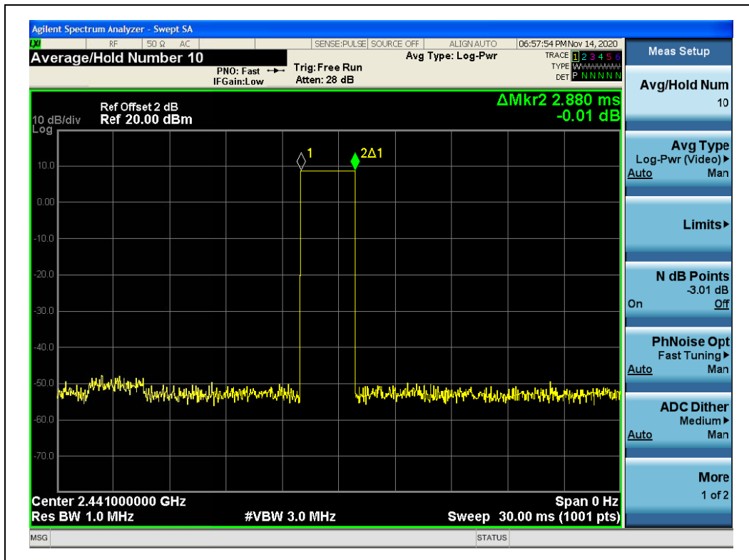
(DH5, GFSK)
