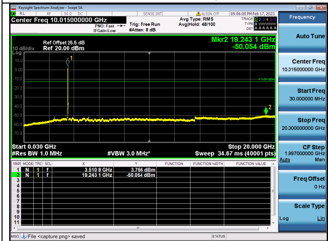
Band42C(3450~3550)-30M-20G / 20MHz+5MHz /100RB+25RB/ QPSK / Mid CH
