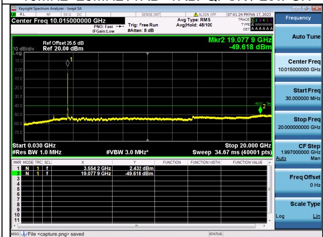
Band42C(3550~3600)-30M-20G / 10MHz+20MHz / 50RB+100RB/ QPSK / Low CH
