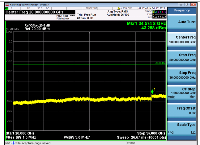
Band42C(3450~3550)-20G-36G / 20MHz+20MHz / 100RB+100RB/ QPSK / Mid CH
