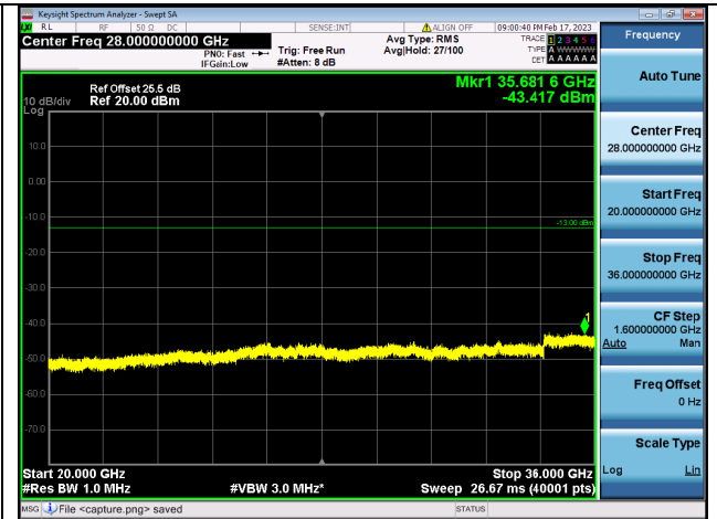
Band42C(3450~3550)-20G-36G / 20MHz+20MHz / 1RB+1RB/ QPSK / Low CH
