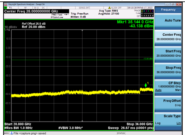
Band42C(3450~3550)-20G-36G / 20MHz+10MHz / 100RB+50RB/ QPSK / Mid CH
