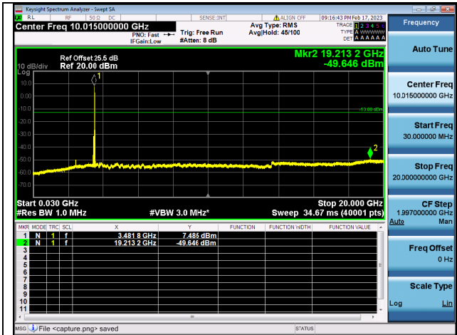
Band42C(3450~3550)-30M-20G / 20MHz+20MHz / 1RB+1RB/ QPSK / Mid CH
