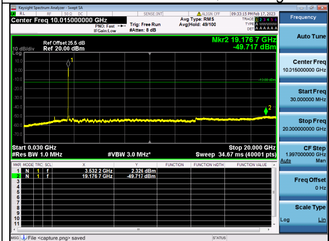
Band42C(3450~3550)-30M-20G / 20MHz+15MHz / 100RB+75RB/ QPSK / High CH
