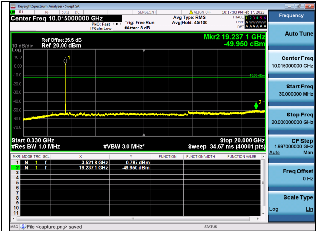
Band42C(3450~3550)-30M-20G / 20MHz+10MHz / 1RB+1RB/ QPSK / High CH
