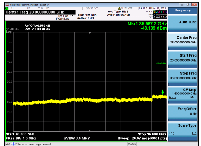
Band42C(3450~3550)-20G-36G / 20MHz+20MHz / 1RB+1RB/ QPSK / Mid CH
