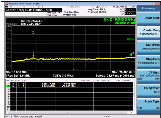
Band42C(3450~3550)-30M-20G / 20MHz+20MHz / 100RB+100RB/ QPSK / Low CH
