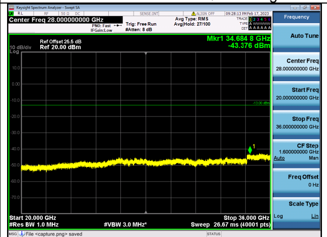
Band42C(3450~3550)-20G-36G / 20MHz+10MHz / 100RB+50RB/ QPSK / High CH
