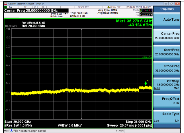
Band42C(3450~3550)-20G-36G / 20MHz+15MHz / 1RB+1RB/ QPSK / Mid CH
