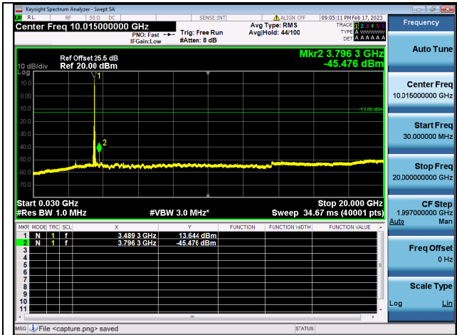
Band42C(3450~3550)-30M-20G / 20MHz+5MHz /1RB+1RB/ QPSK / Mid CH
