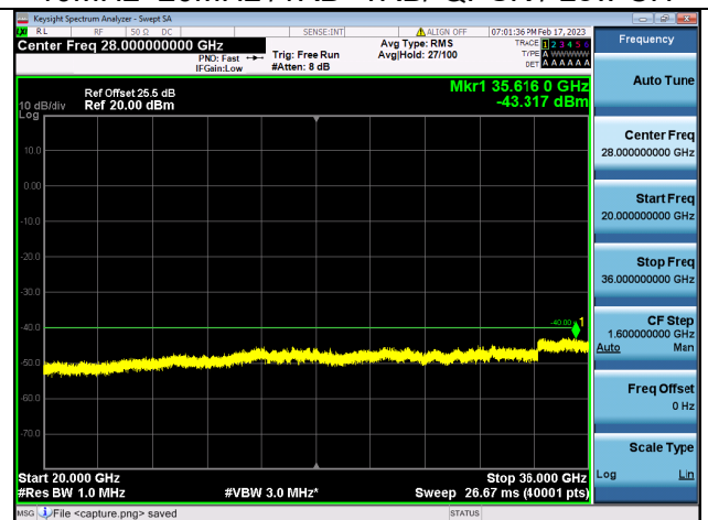
Band42C(3550~3600)-20G-36G / 10MHz+20MHz / 50RB+100RB/ QPSK / Low CH
