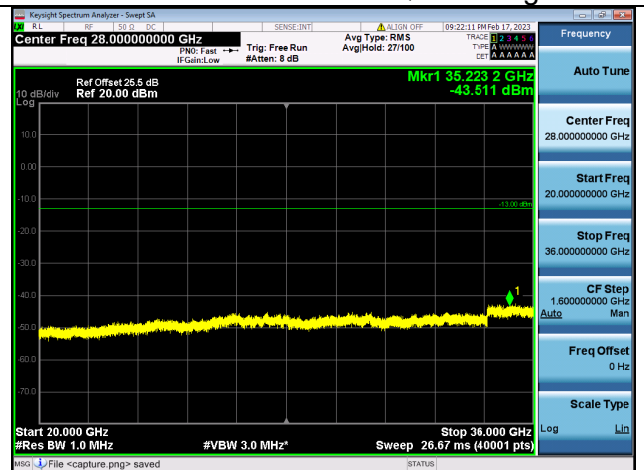
Band42C(3450~3550)-20G-36G / 20MHz+5MHz / 100RB+25RB/ QPSK / High CH
