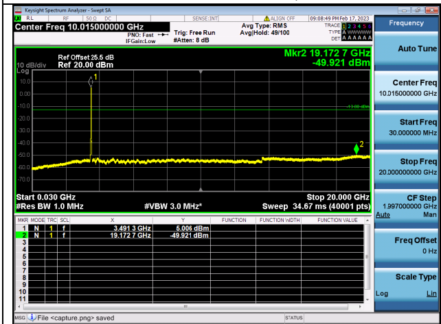
Band42C(3450~3550)-30M-20G / 10MHz+20MHz / 50RB+100RB/ QPSK / Mid CH
