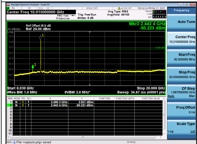
Band42C(3450~3550)-30M-20G / 20MHz+15MHz / 100RB+75RB/ QPSK / Mid CH
