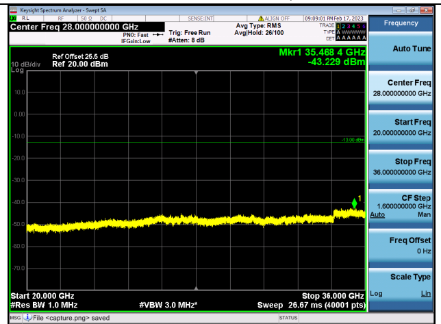
Band42C(3450~3550)-20G-36G / 10MHz+20MHz / 50RB+100RB/ QPSK / Mid CH
