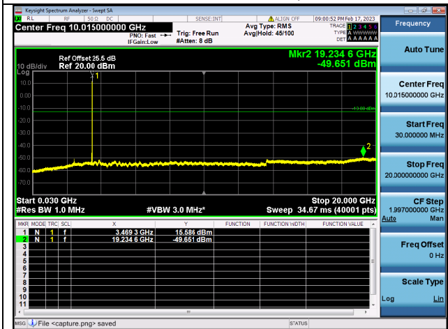
Band42C(3450~3550)-30M-20G / 20MHz+20MHz / 1RB+1RB/ QPSK / Low CH
