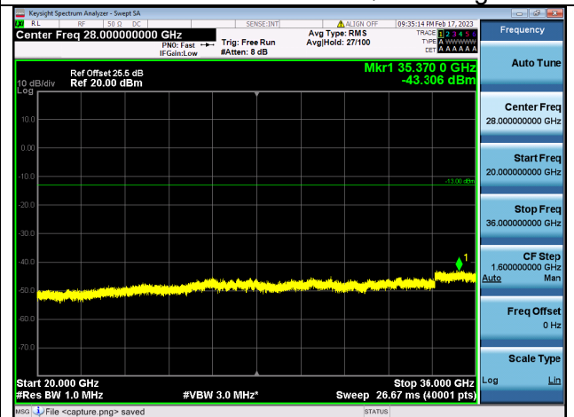
Band42C(3450~3550)-20G-36G / 20MHz+20MHz / 1RB+1RB/ QPSK / High CH
