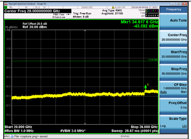
Band42C(3450~3550)-20G-36G / 20MHz+10MHz / 1RB+1RB/ QPSK / Mid CH
