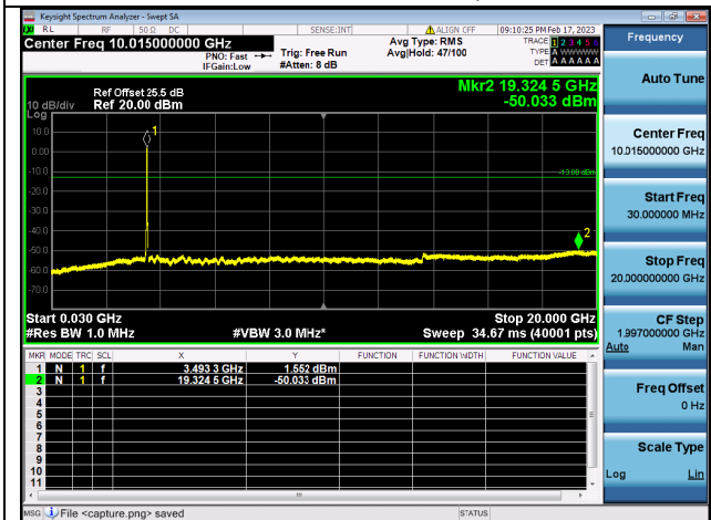
Band42C(3450~3550)-30M-20G / 20MHz+10MHz / 100RB+50RB/ QPSK / Mid CH
