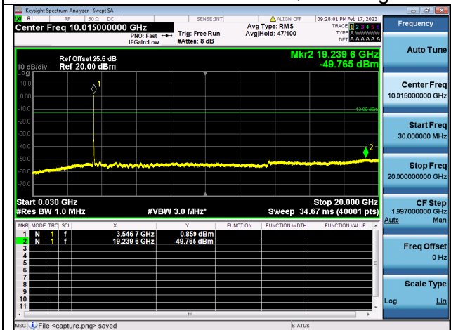
Band42C(3450~3550)-30M-20G / 20MHz+10MHz / 100RB+50RB/ QPSK / High CH
