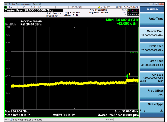
Band42C(3450~3550)-20G-36G / 10MHz+20MHz / 1RB+1RB/ QPSK / High CH
