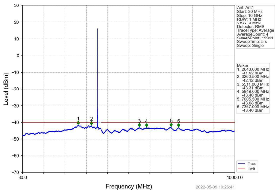
Band48_10MHz_QPSK_LCH_3555MHz_RB_1_0_NTNV
