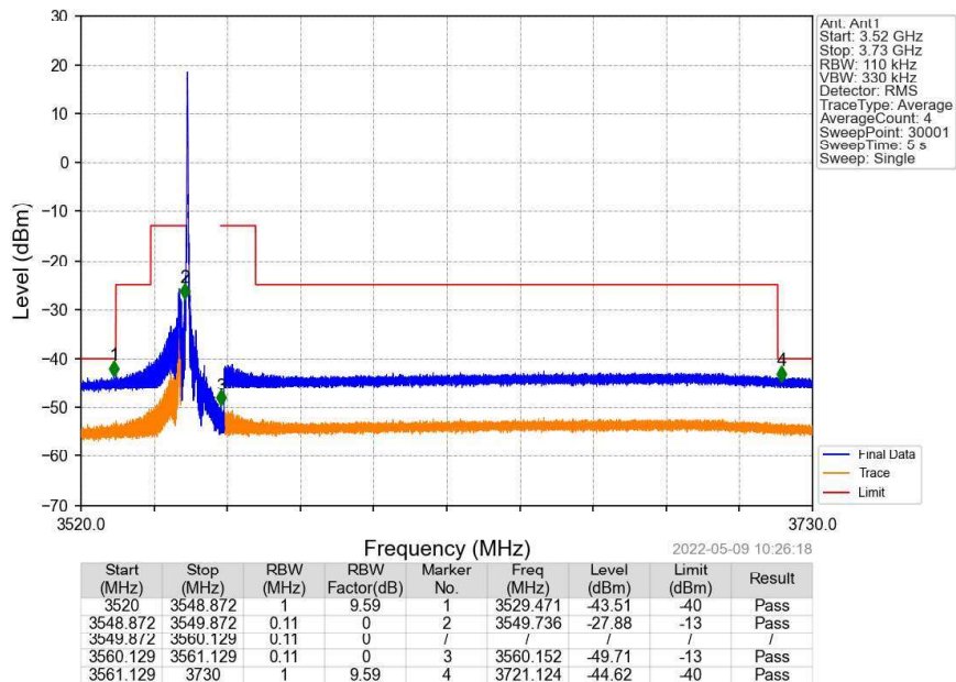
Band48_10MHz_QPSK_LCH_3555MHz_RB_1_0_NTNV
