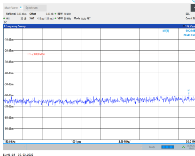
Band13-10MHz-QPSK-23230-1RB#0-Range2:0.15~30MHz
