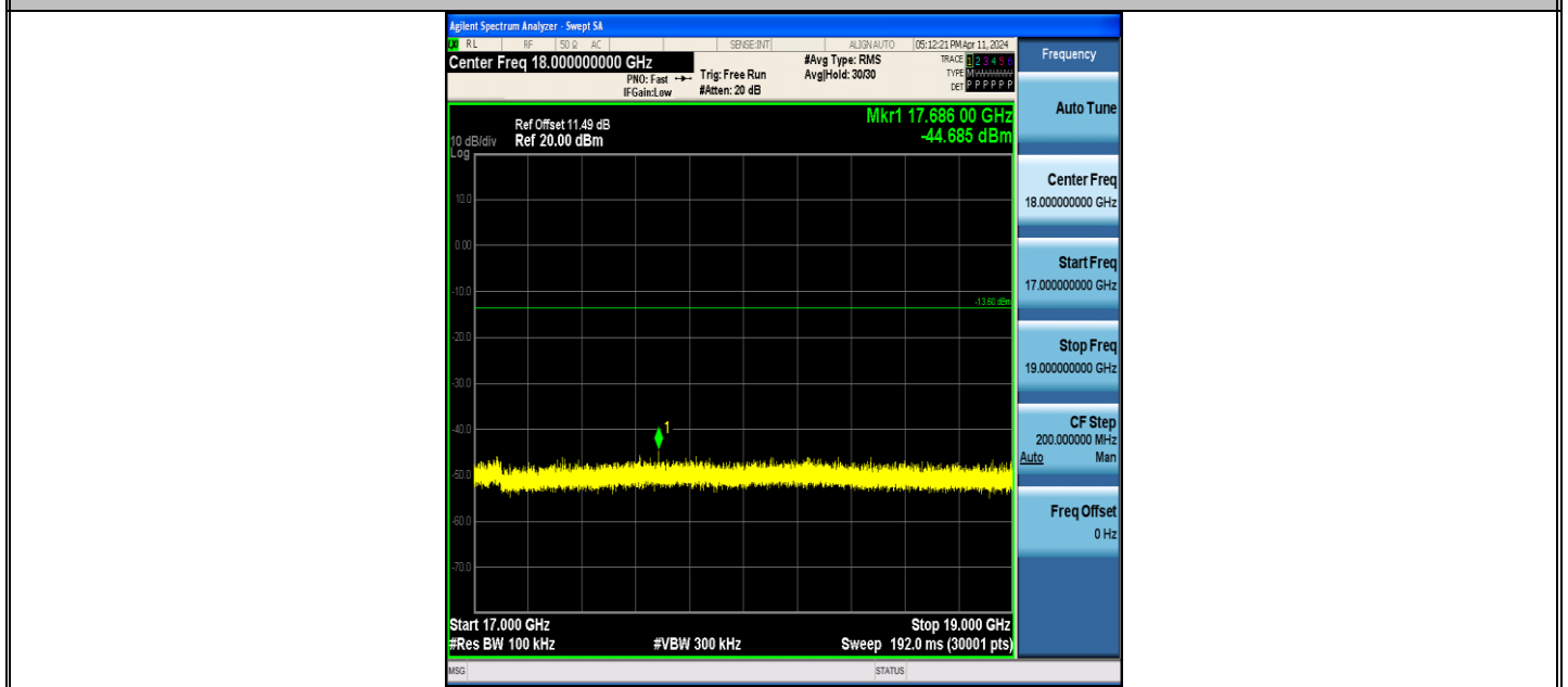
BLE_125K-Ant1-2480-17000~19000-PASS
