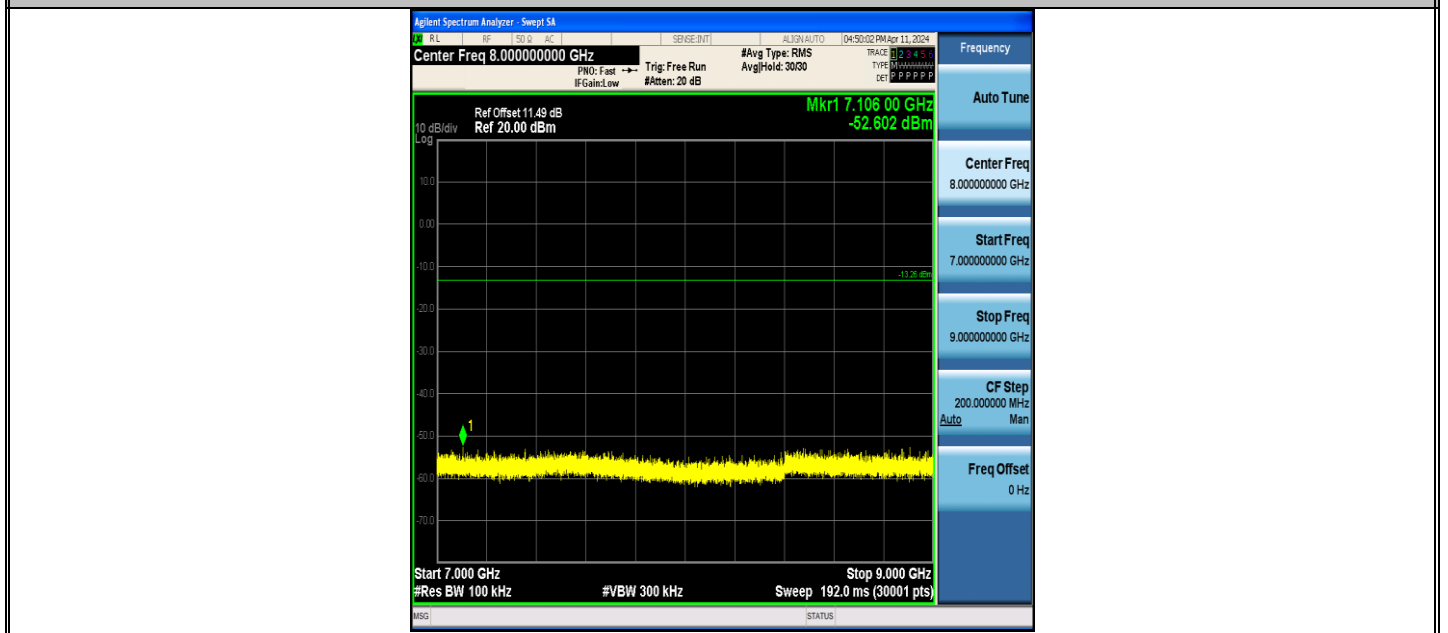
BLE_2M-Ant1-2480-7000~9000-PASS
