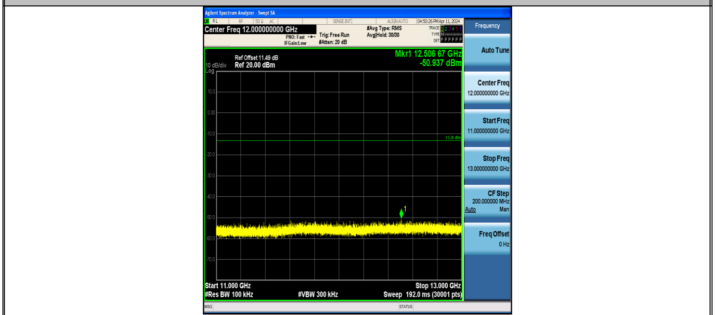
BLE_2M-Ant1-2480-11000~13000-PASS
