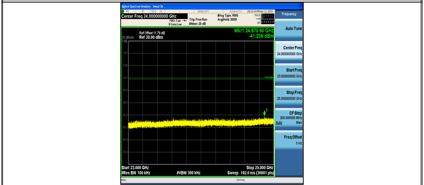
BLE_500K-Ant1-2402-23000~25000-PASS
