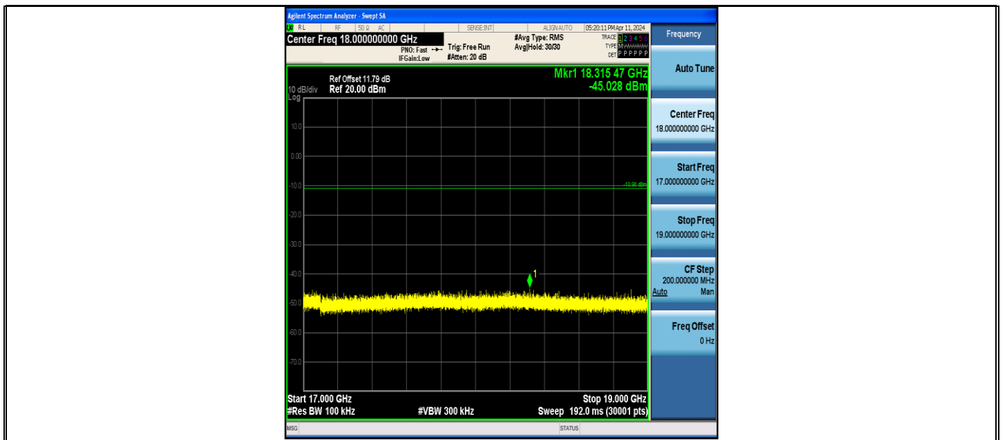
BLE_500K-Ant1-2402-17000~19000-PASS
