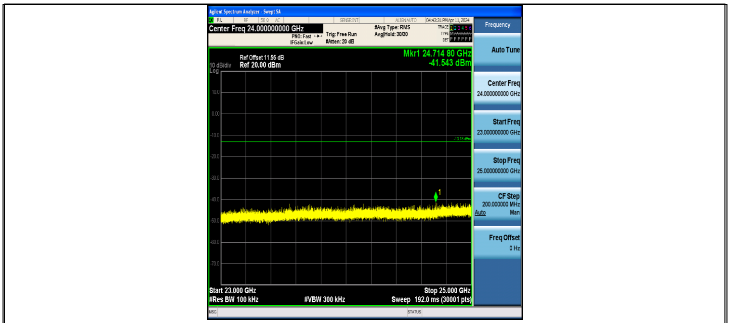
BLE_2M-Ant1-2440-23000~25000-PASS
