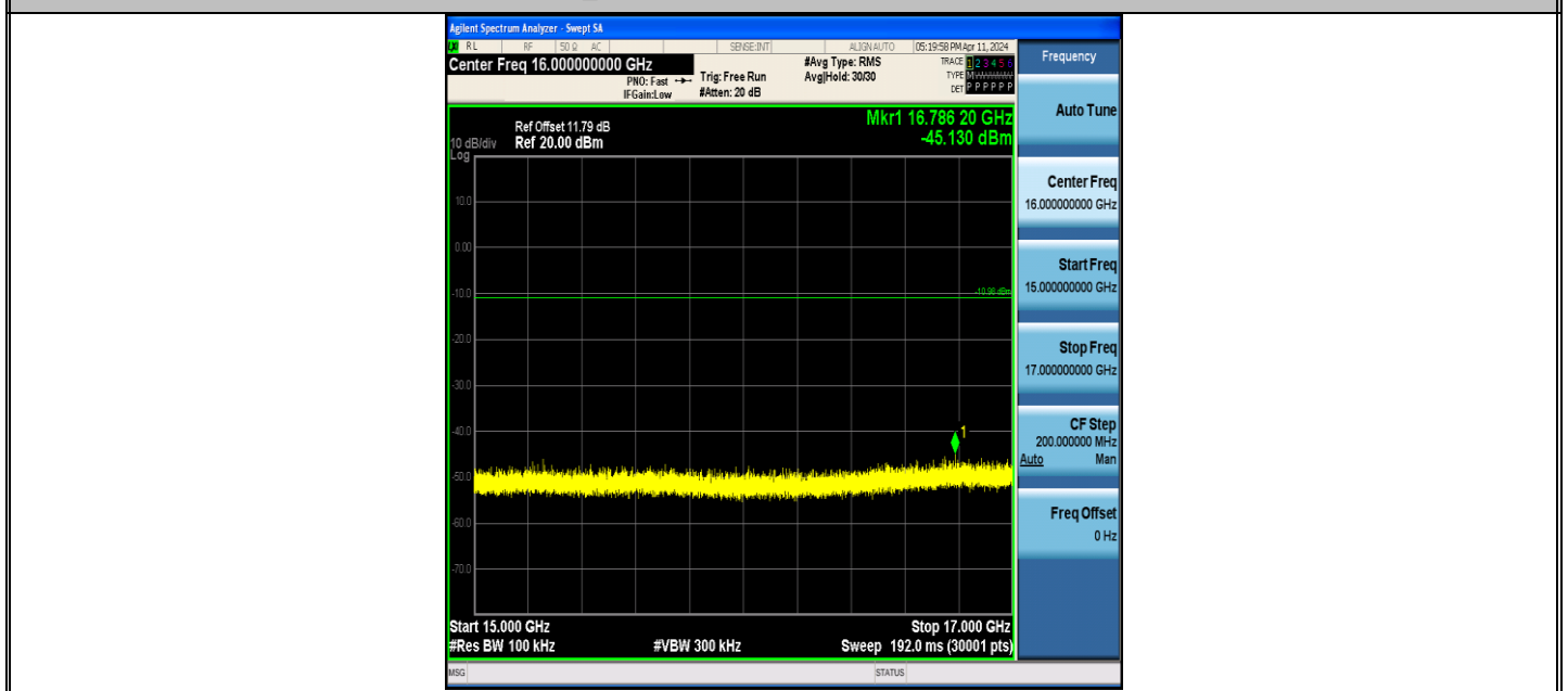
BLE_500K-Ant1-2402-15000~17000-PASS
