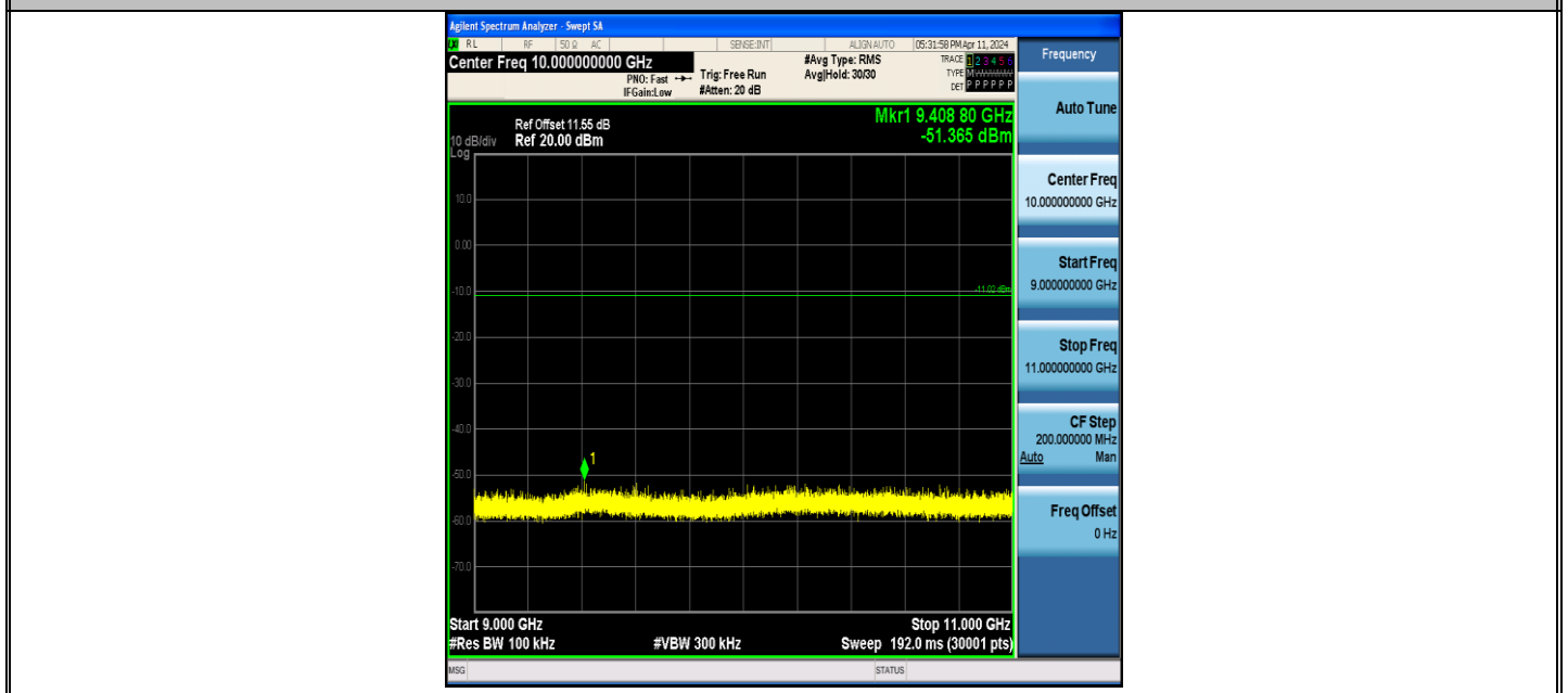
BLE_500K-Ant1-2440-9000~11000-PASS
