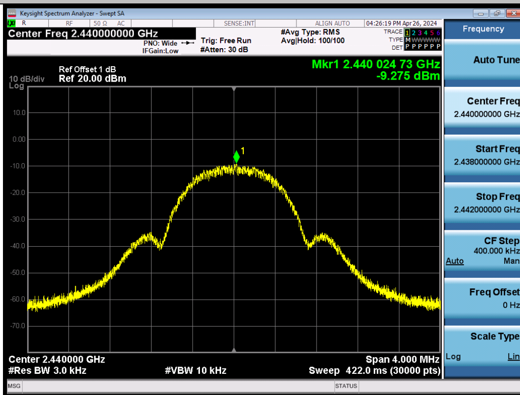
BLE_500K-Ant1-2440-PASS
