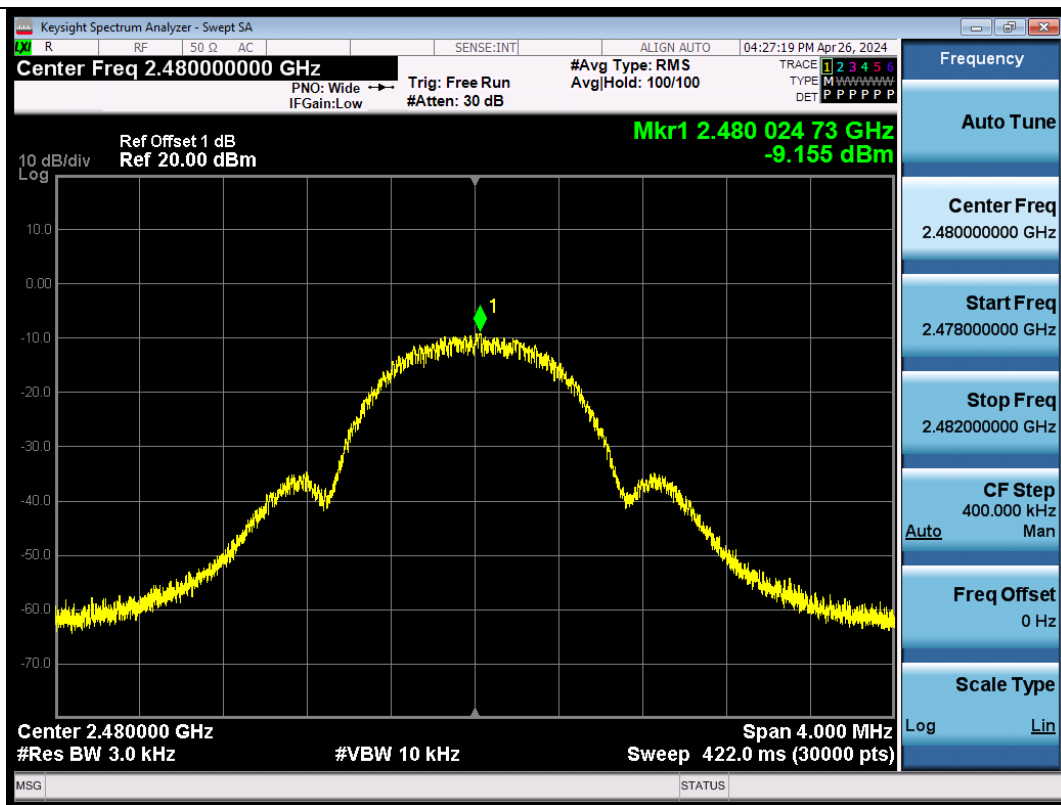
BLE_500K-Ant1-2480-PASS
