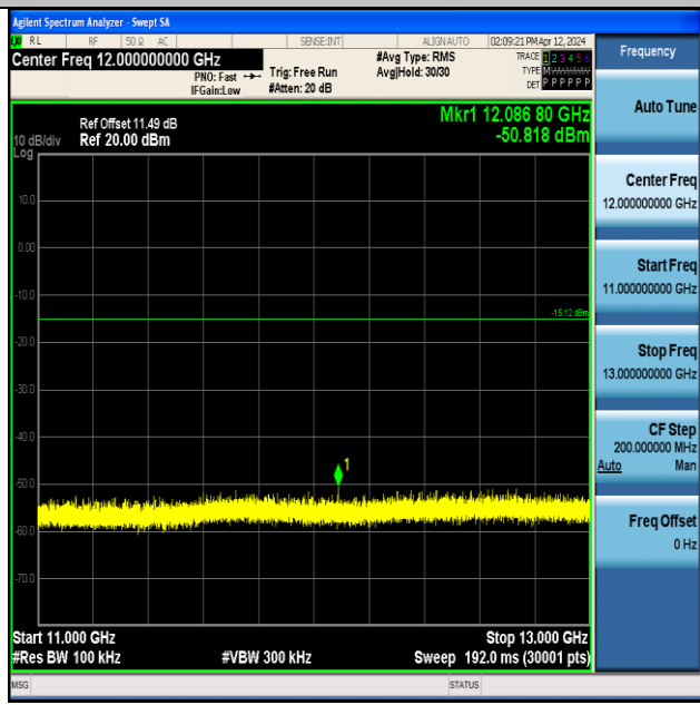
BLE_2M-Ant1-2480-11000~13000-PASS
