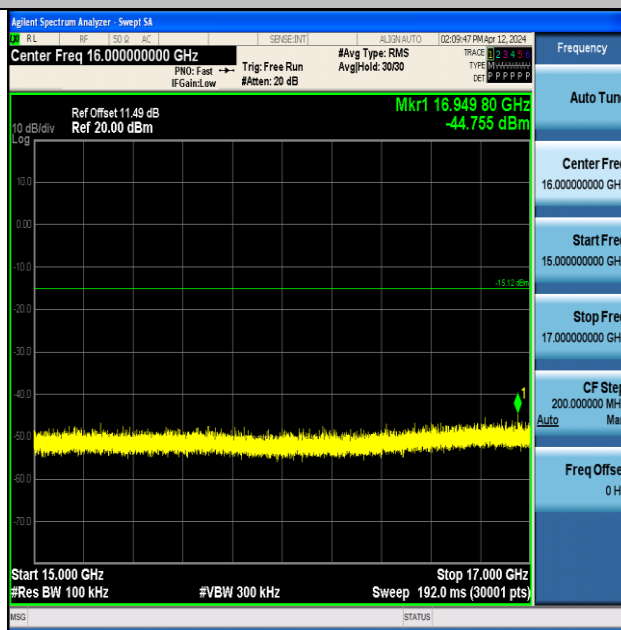
BLE_2M-Ant1-2480-15000~17000-PASS
