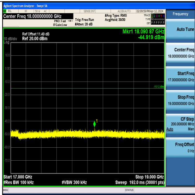
BLE_2M-Ant1-2480-17000~19000-PASS
