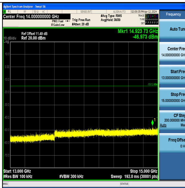
BLE_2M-Ant1-2480-13000~15000-PASS
