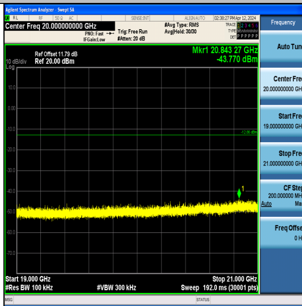
BLE_500K-Ant1-2402-19000~21000-PASS
