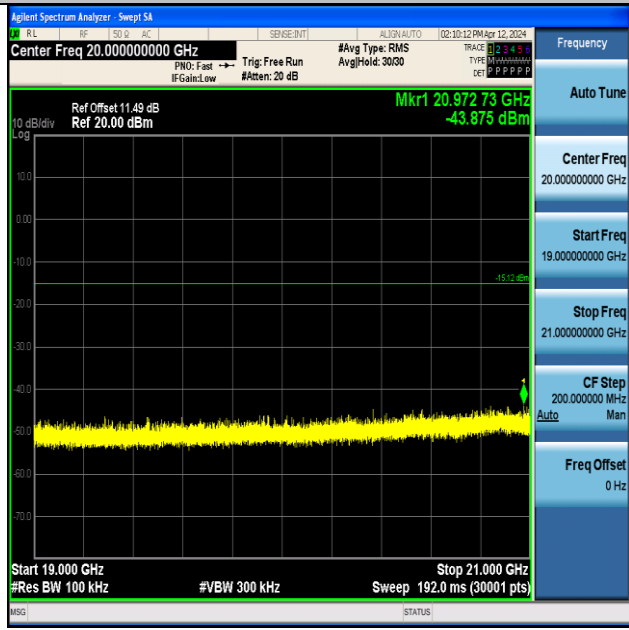
BLE_2M-Ant1-2480-19000~21000-PASS
