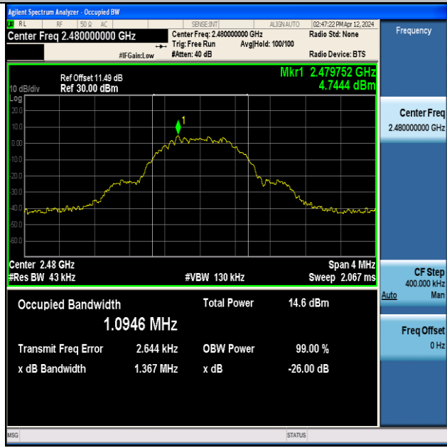
BLE_500K-Ant1-2480
