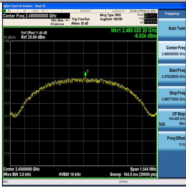
BLE_500K-Ant1-2480-PASS
