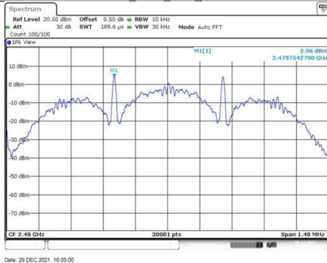
BLE 125K_Ant1_2480
