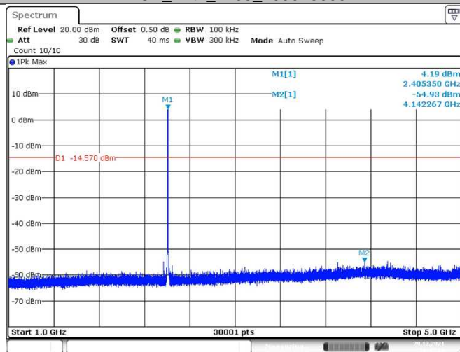
ZIGB_Ant1_2405_1000~5000
