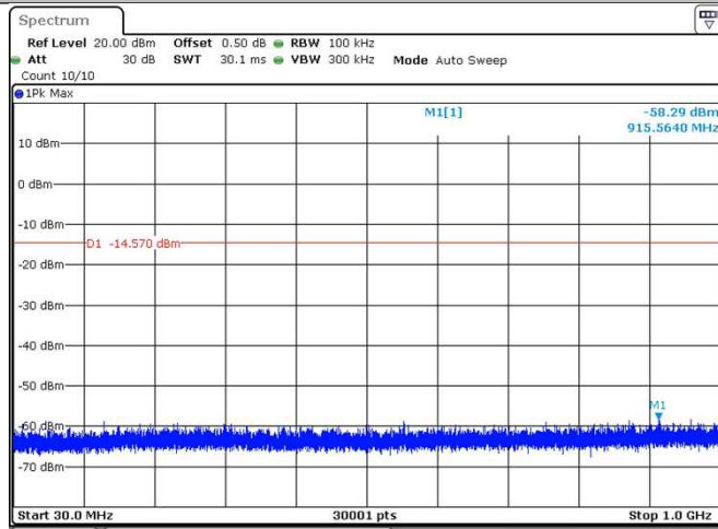
ZIGB_Ant1_2405_30~1000
