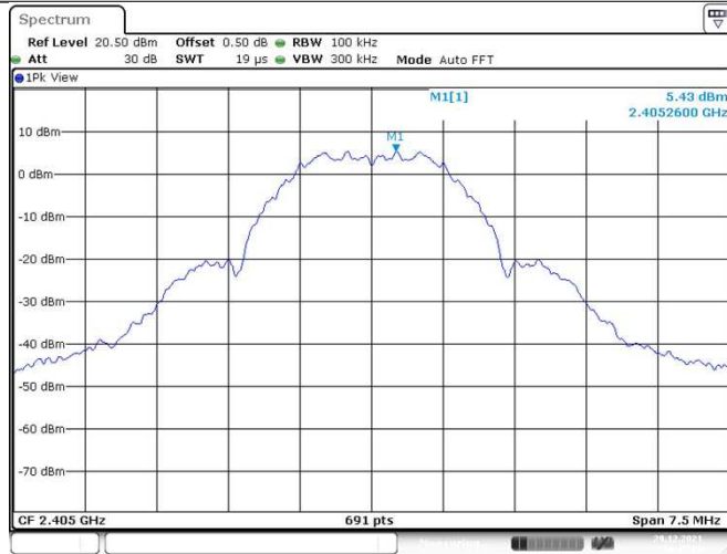
ZIGB_Ant1_2405_0~Reference
