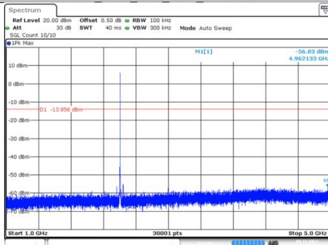
BLE_125K_Ant1_2402_1000~5000
