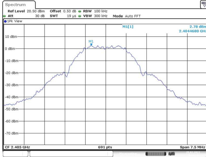
ZIGB_Ant1_2405_0~Reference
