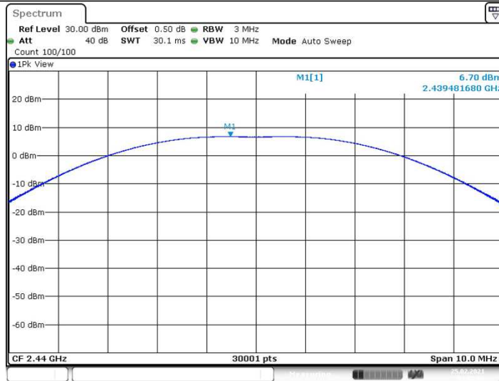
ZIGB_Ant1_2440
