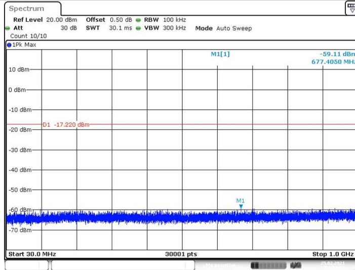
ZIGB_Ant1_2405_30~1000
