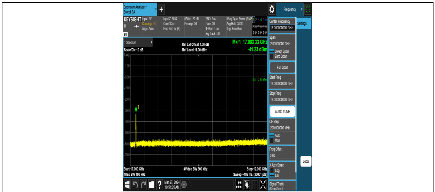
ZIGB-Ant1-2440-17000~19000-PASS
