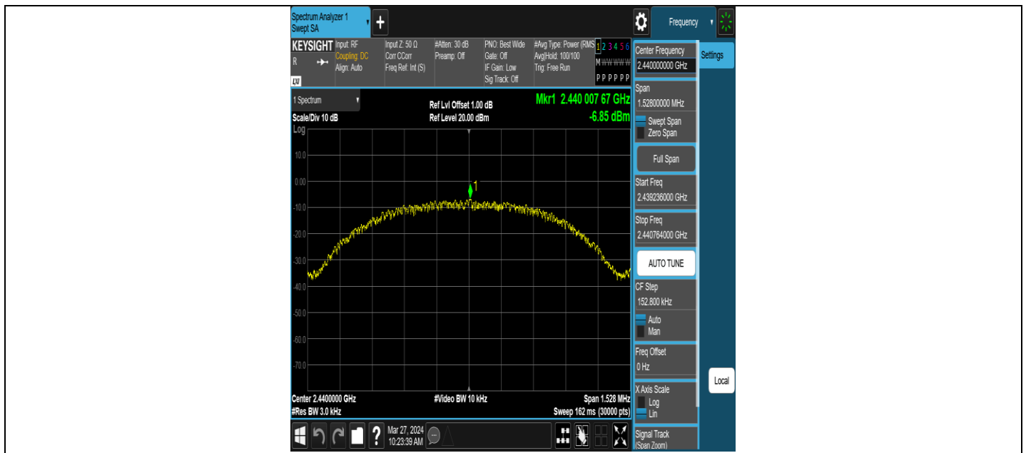
BLE_500K-Ant1-2440-PASS
