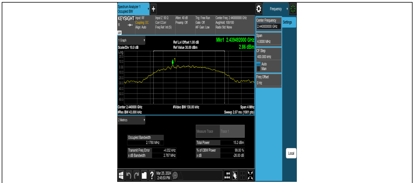
BLE_2M-Ant1-2440
