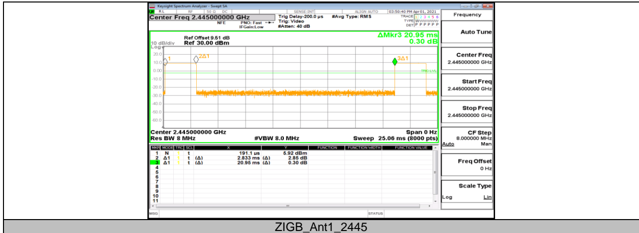
ZIGB_Ant1_2445
