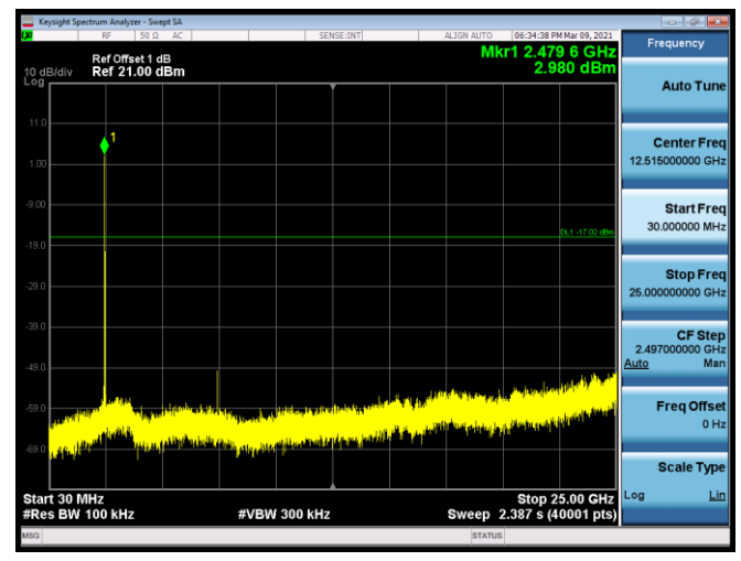
Mode1/CH26/2480MHz
