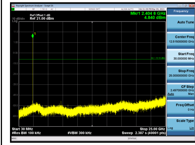
Mode1/CH11/2405MHz
