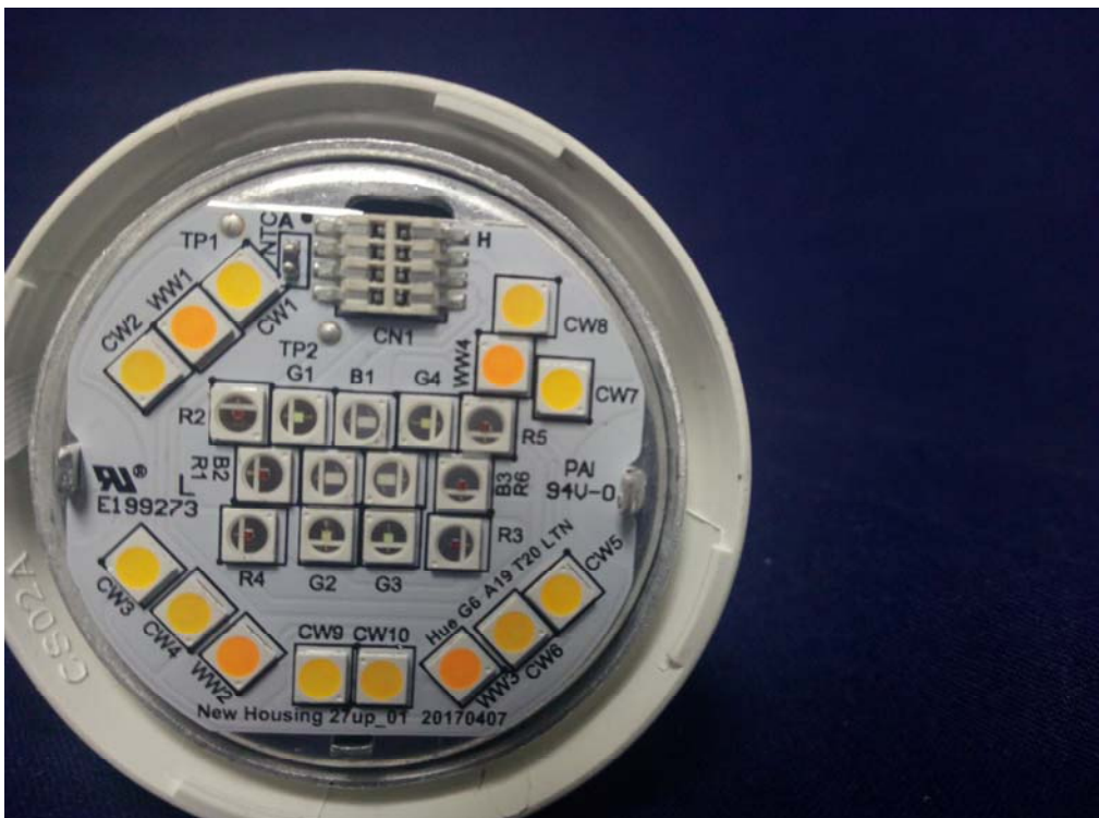
(10) EUT Photo(LTN+Alvis+Diodes)
