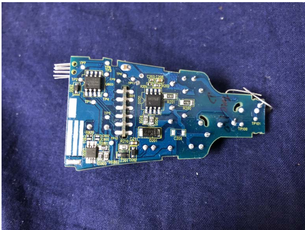
(2) EUT Photo(Alvis+Diodes)
