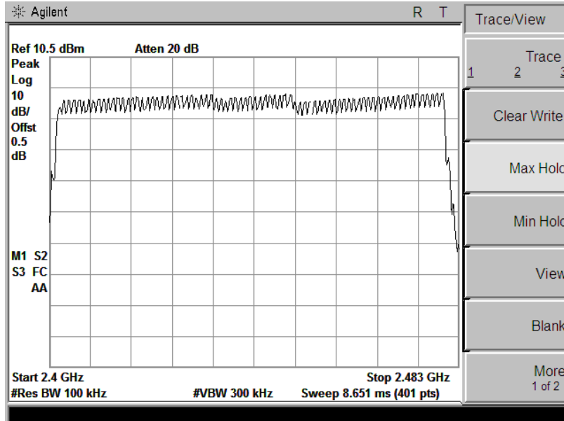
8DPSK Mode
