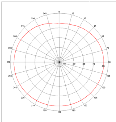
XY-plane
