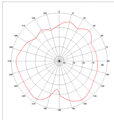
XZ-plane
