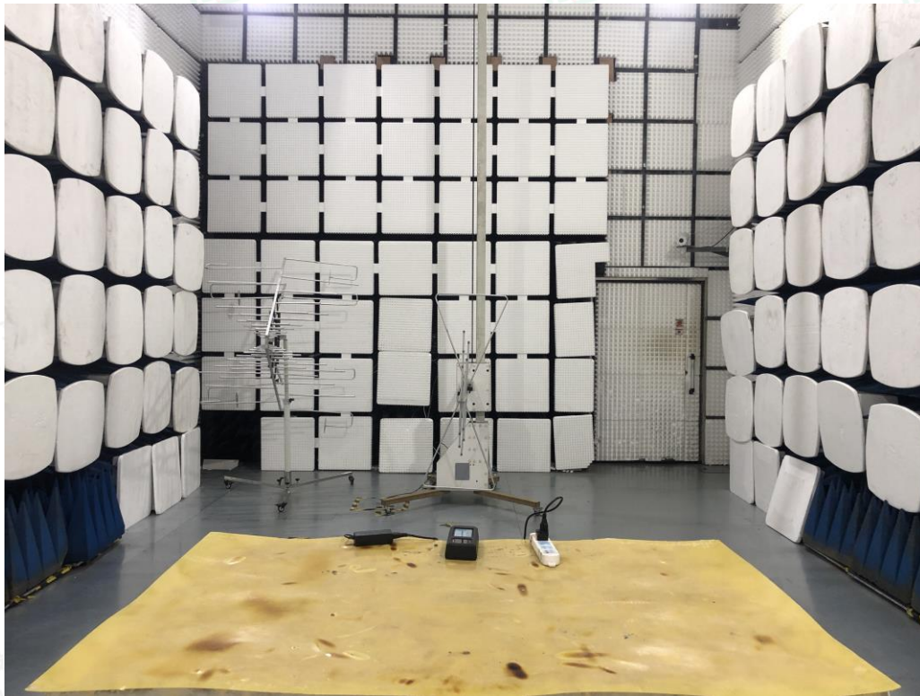
Fig. 2 (30MHz~1GHz)
