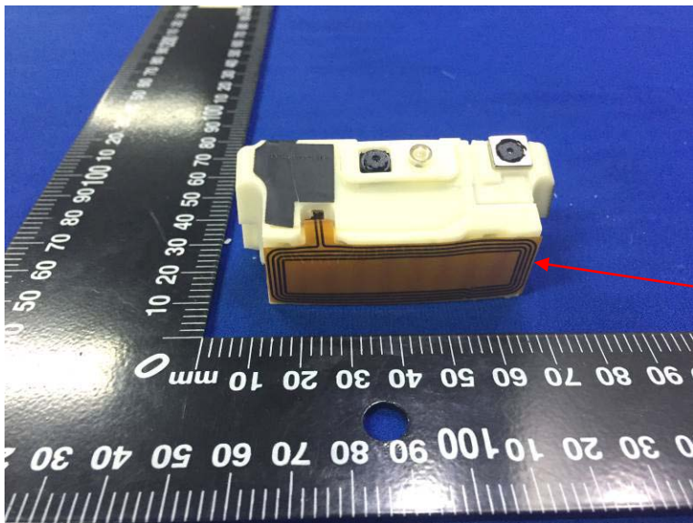
RFID Antenna
