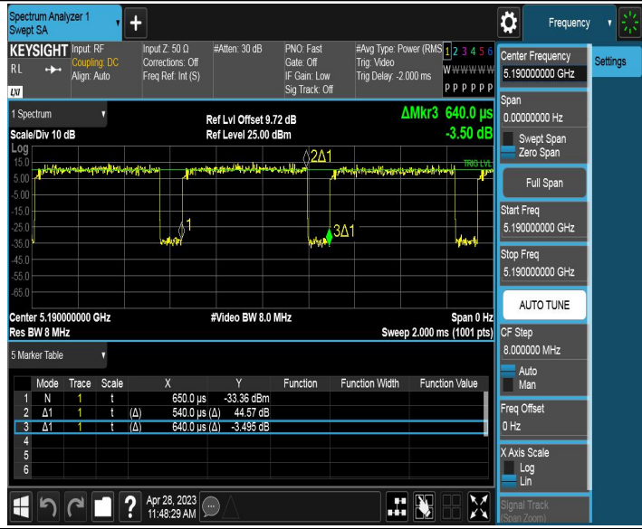
11AX40MIMO_Ant2_5190
