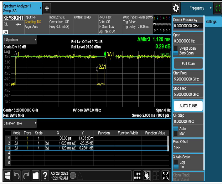
11AX20MIMO_Ant2_5200
