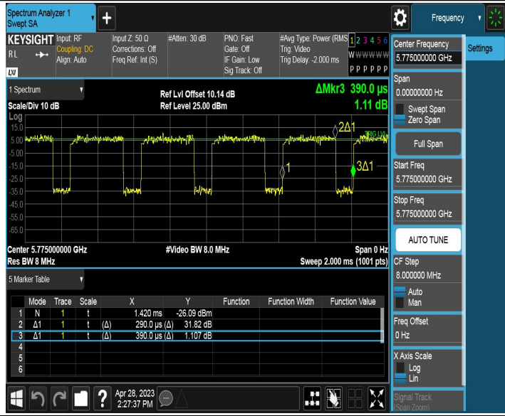
11AX80MIMO_Ant2_5775
