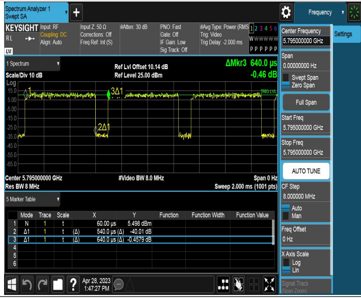
11AX40MIMO_Ant1_5795
