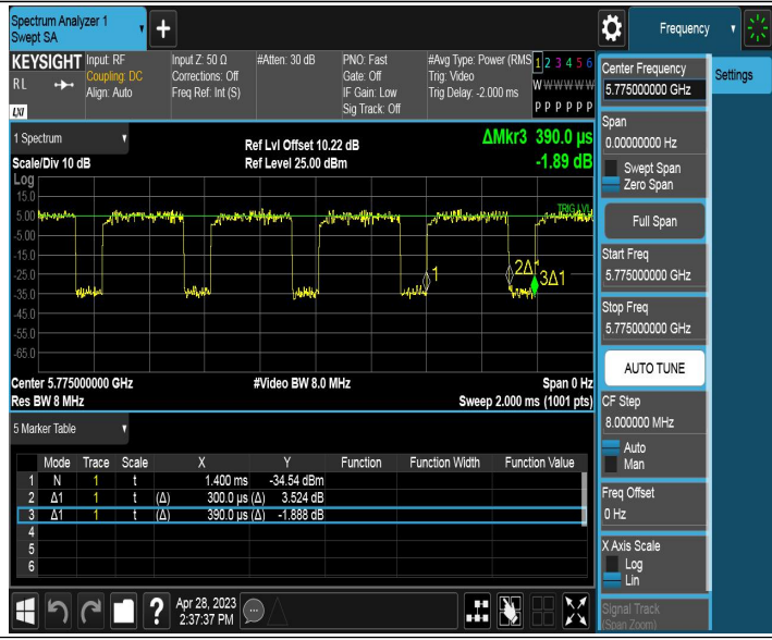
11AX80MIMO_Ant2_5775
