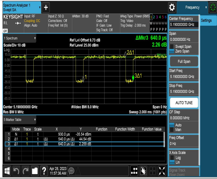
11AX40MIMO_Ant2_5190
