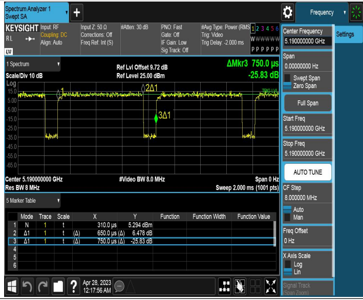
11AC40MIMO_Ant1_5190
