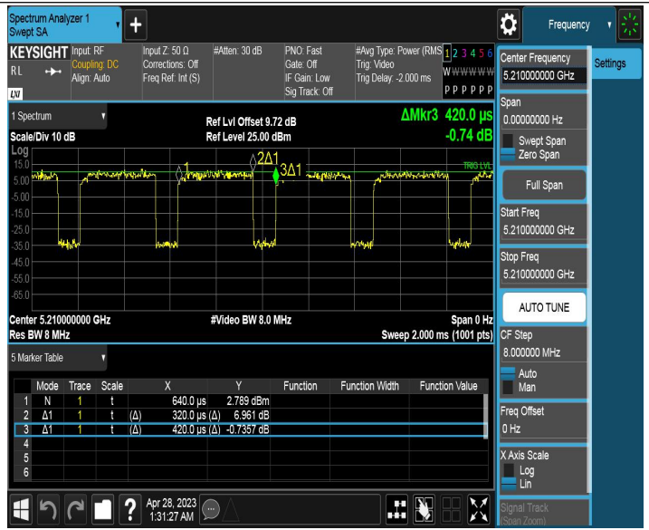
11AC80MIMO_Ant2_5210
