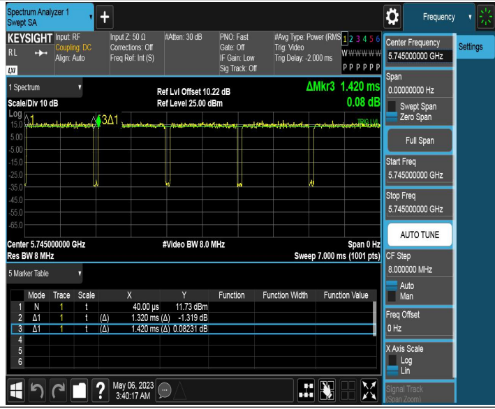
11AC20MIMO_Ant2_5745
