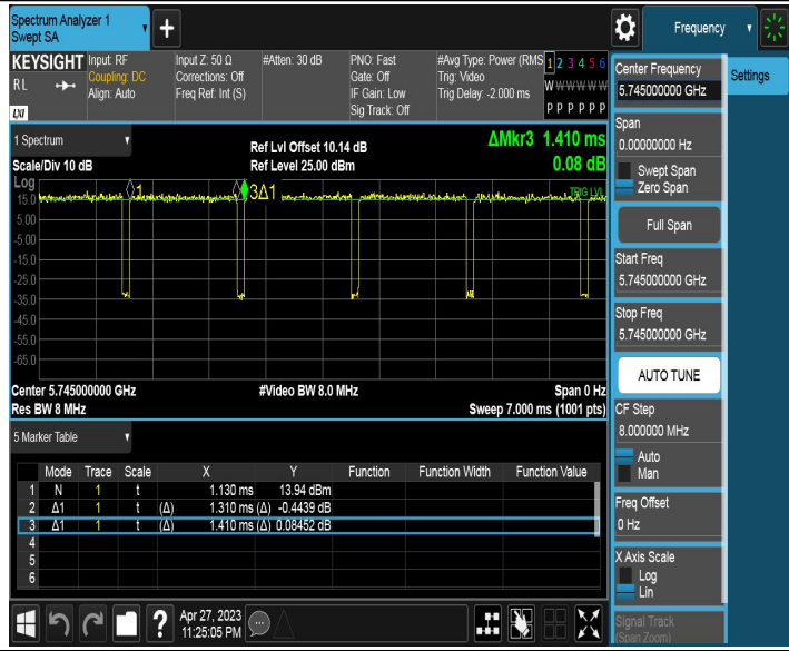
11AC20MIMO_Ant2_5745
