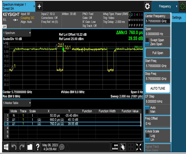
11AC40MIMO_Ant1_5755
