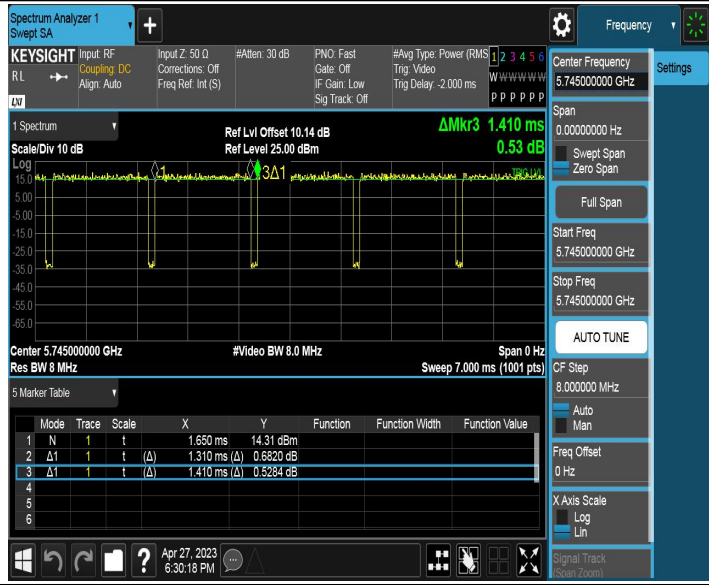
11N20MIMO_Ant2_5745
