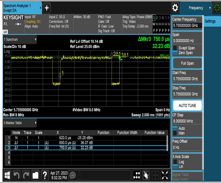
11N40MIMO_Ant2_5755
