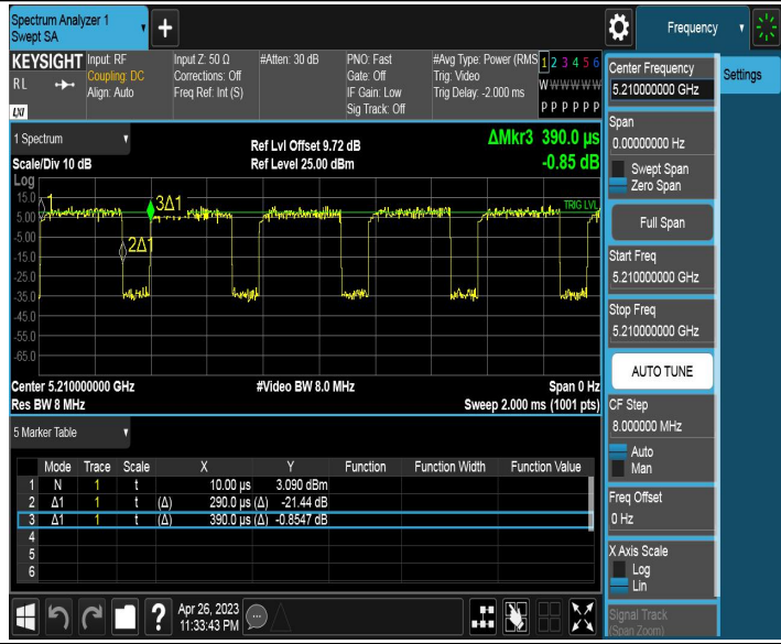
11AX80SISO_Ant2_5210
