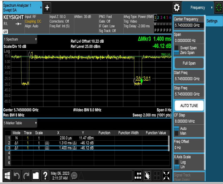
11N20MIMO_Ant2_5745
