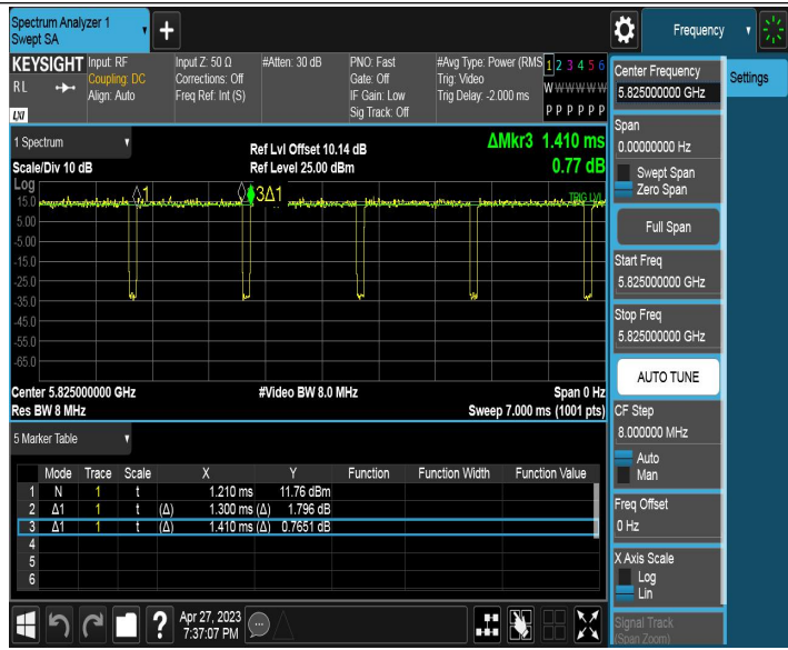
11N20MIMO_Ant2_5825
