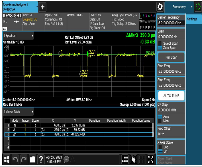
11AX80SISO_Ant2_5210
