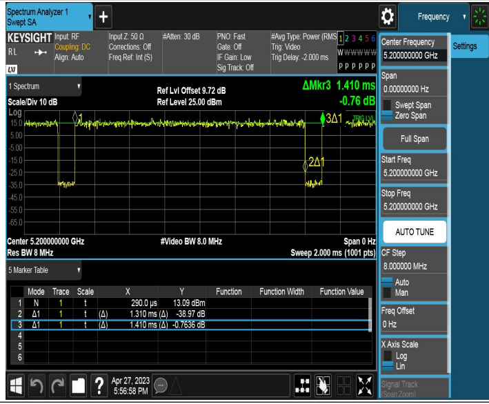
11N20MIMO_Ant1_5200
