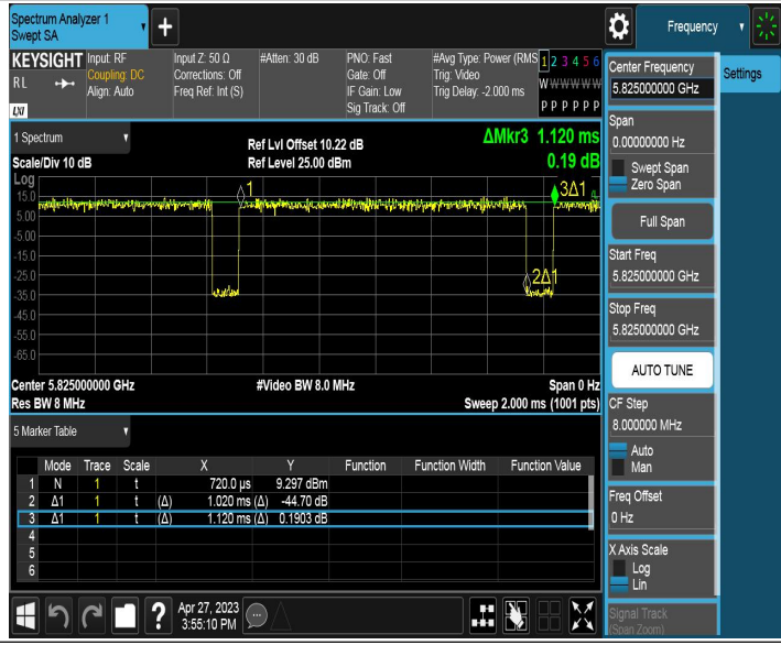
11AX20SISO_Ant2_5825
