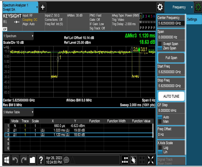
11AX20SISO_Ant2_5825
