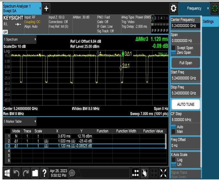
11AX20SISO_Ant2_5240
