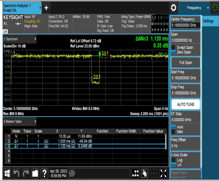
11AX20SISO_Ant2_5180
