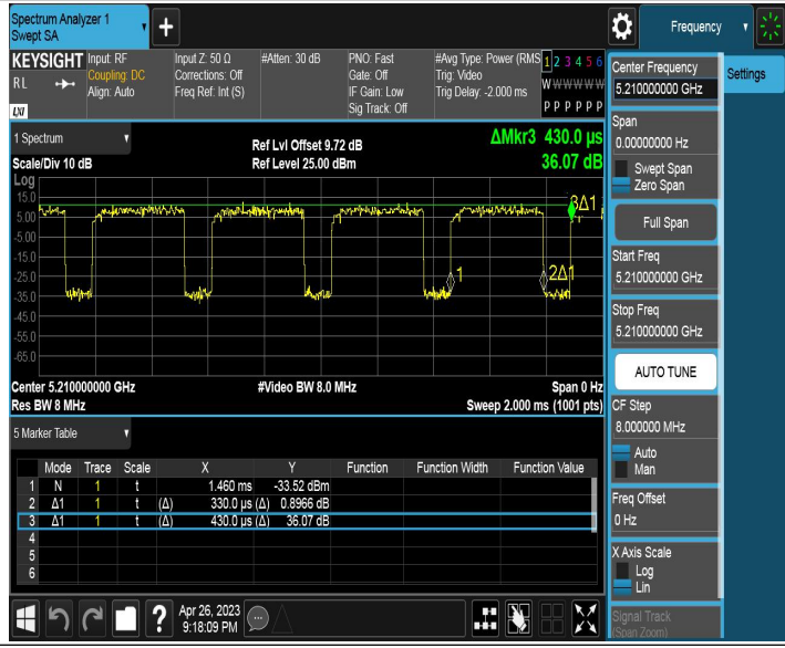
11AC80SISO_Ant1_5210
