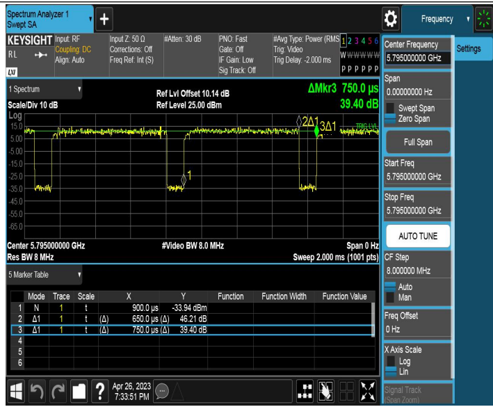
11N40SISO_Ant2_5795
