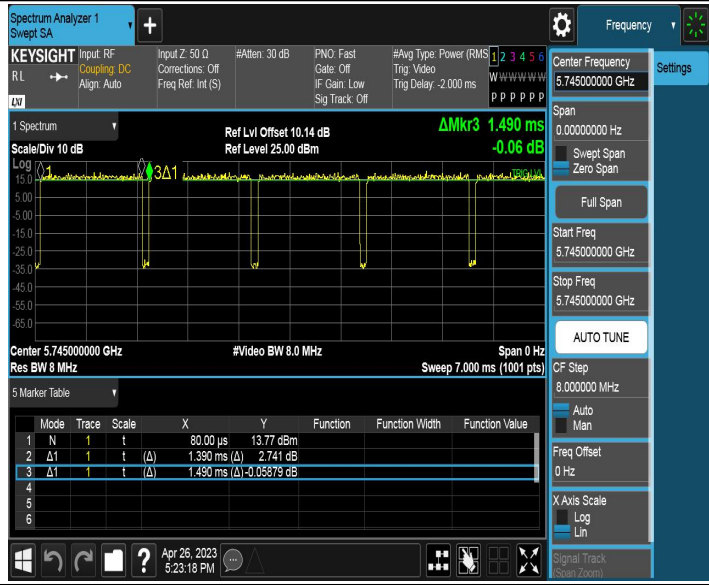
11A_Ant2_5745
