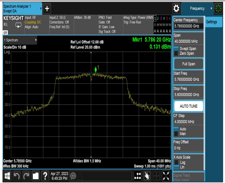
11N20MIMO_Ant2_5785
