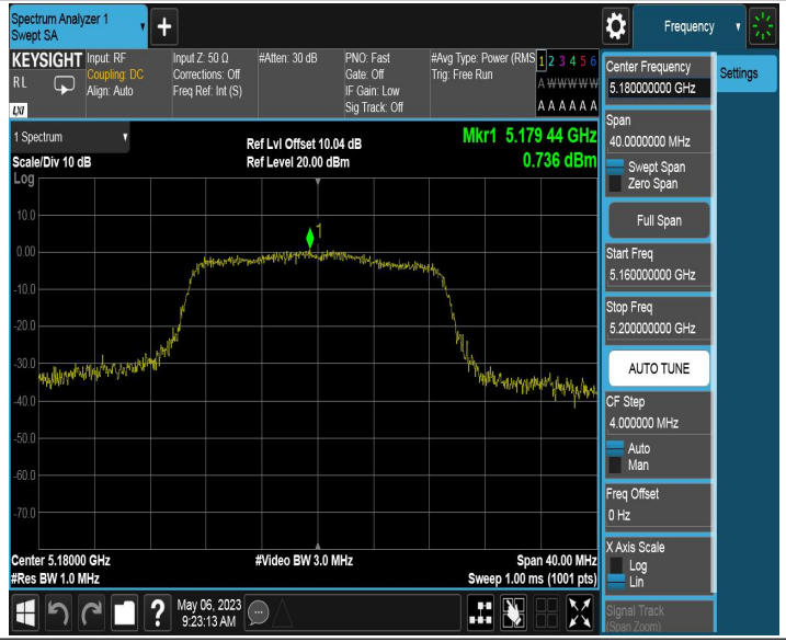
11AC20MIMO_Ant1_5180
