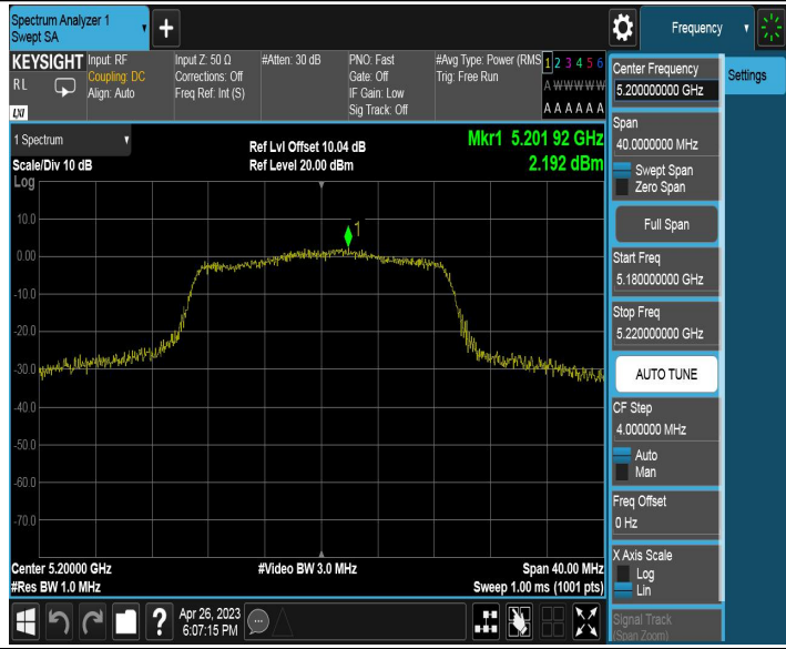
11N20SISO_Ant2_5200
