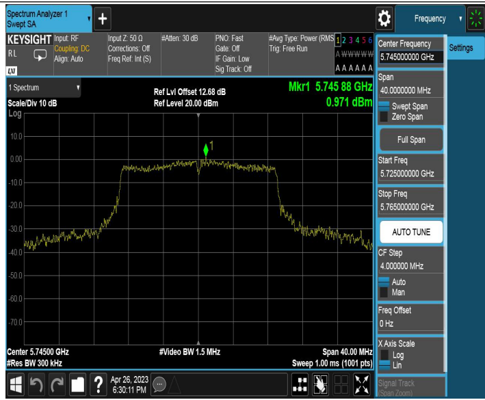
11N20SISO_Ant2_5745
