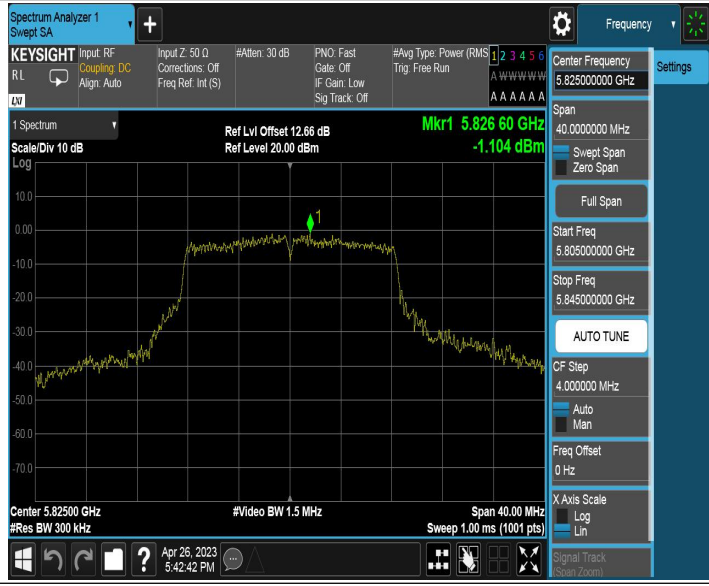
11A_Ant1_5825
