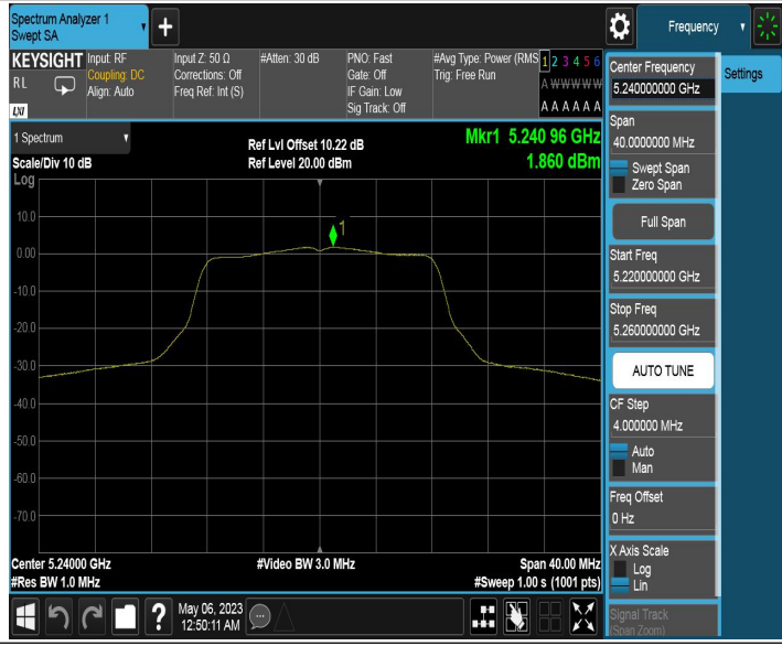
11A_Ant2_5240
