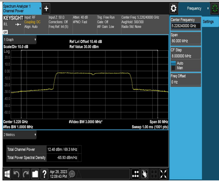
11AX40MIMO_Ant2_5230
