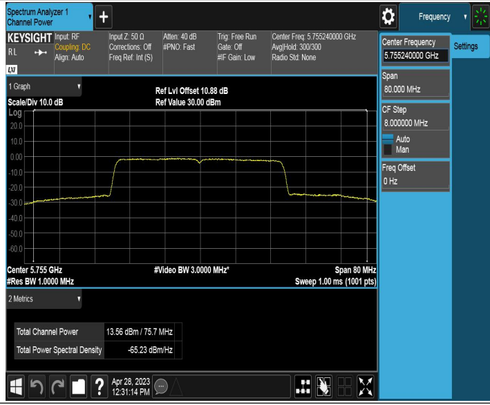
11AX40MIMO_Ant1_5755
