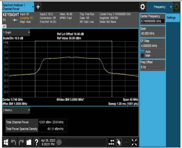
11N20SISO_Ant2_5745
