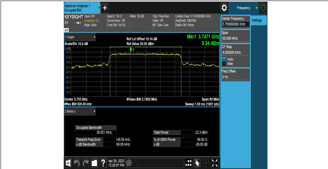
11AX40MIMO_Ant2_5755
