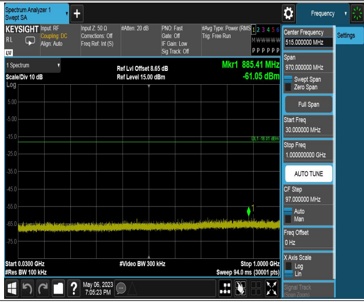
11AX20SISO_Ant1_2462_30~1000
