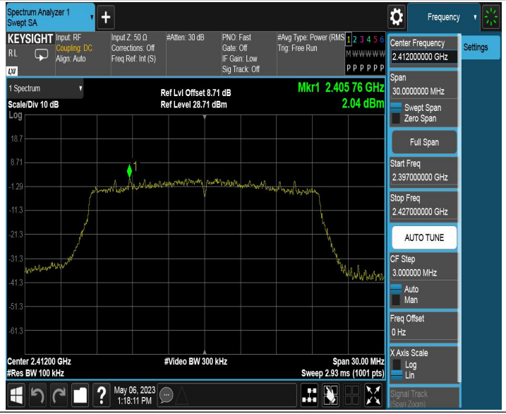
11AX20MIMO_Ant1_2412_0~Reference
