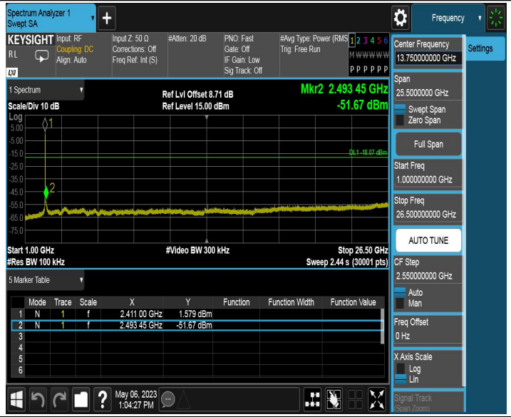
11AX20SISO_Ant2_2412_0~Reference
