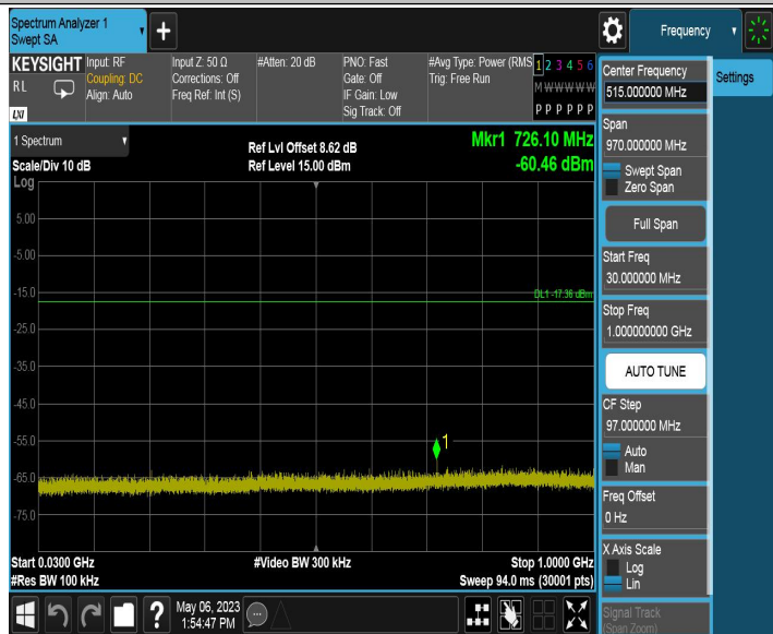
11AX20MIMO_Ant2_2437_30~1000
