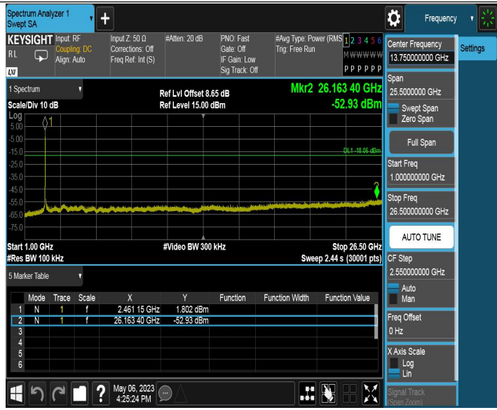
11N20MIMO_Ant2_2462_0~Reference
