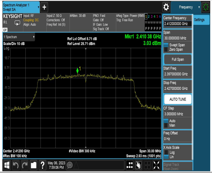
11AX20SISO_Ant2_2412_0~Reference
