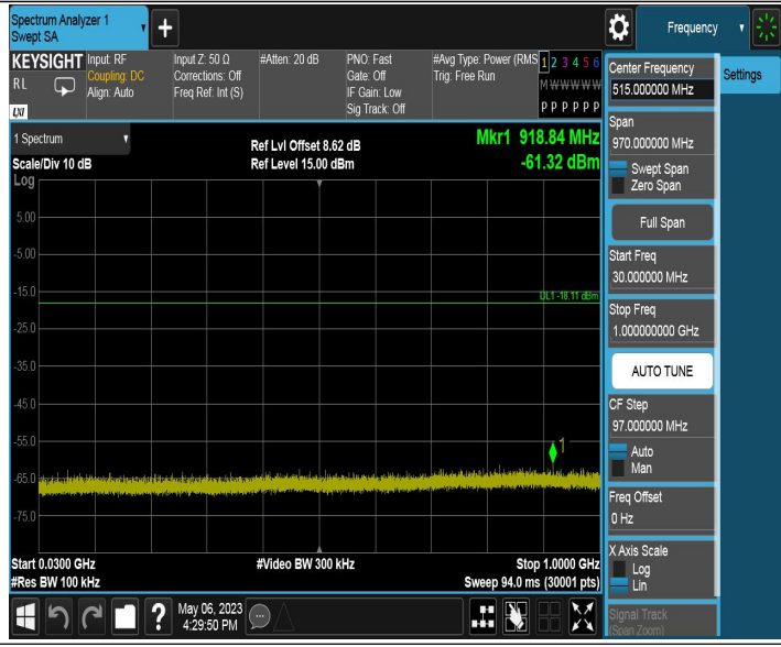
11N20MIMO_Ant2_2462_30~1000
