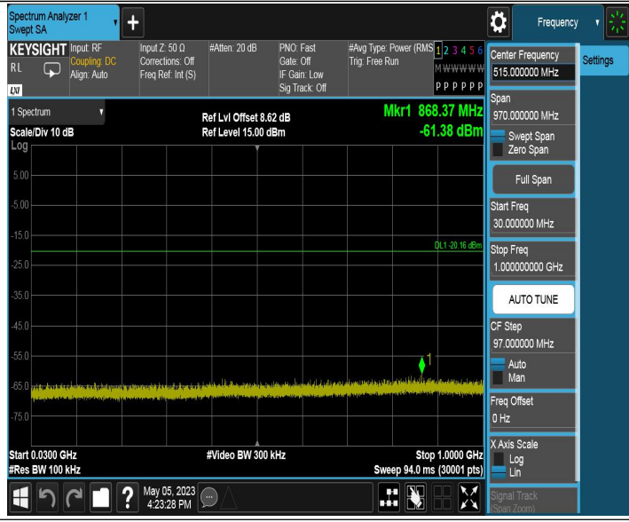
11G_Ant2_2462_30~1000
