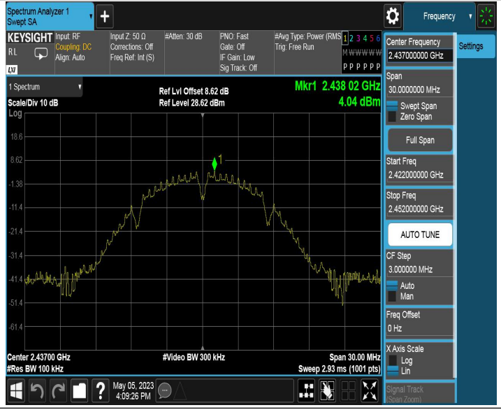
11B_Ant2_2437_0~Reference
