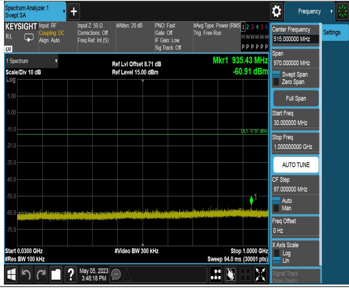
11G_Ant1_2412_30~1000
