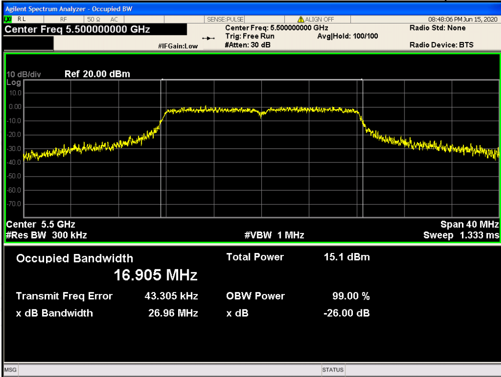
OBW NVNT 802.11a 5600MHz Ant0
