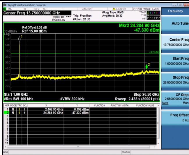
11G_Ant1_2462_1000~26500
