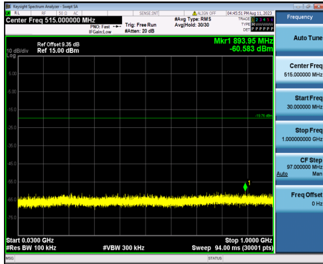
11G_Ant1_2462_30~1000
